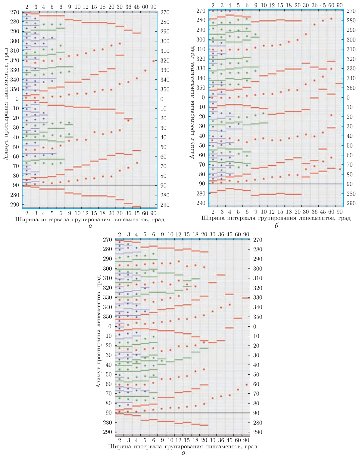
Рис. 1. Графики выделения систем линеаментов при разной ширине интервала группирования: a — Тарханкутский полуостров, Крым; b — район Чернобыльской АЭС; v — юго-восточная часть Днепро-Донецкой впадины. Условные обозначения. Красные линии — системы линеаментов максимальной протяженности (ширина интервала группирования 2–90°); зеленые линии — системы линеаментов средней протяженности (ширина интервала группирования 2–20°); синие линии — системы линеаментов минимальной протяженности (ширина интервала группирования 2–5°). Звездочки — модальные значения системы линеаментов
