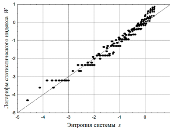
Рисунок 1 – Зависимость статистического индекса ( W ) от энтропии системы ( s ) для распределения совместно наблюдаемых значений атрибутивных величин ( \rho_2, \rho_4, \rho_5 ) для 177 стран мира
