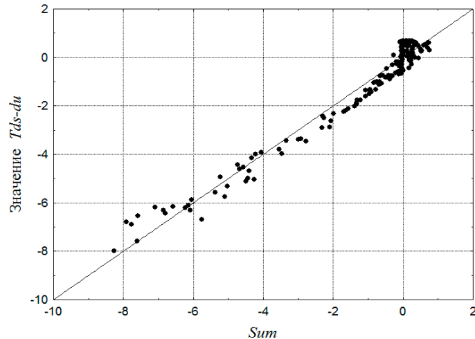
Рисунок 2 – Обработка данных для уравнения (10) относительно опорного состояния:
