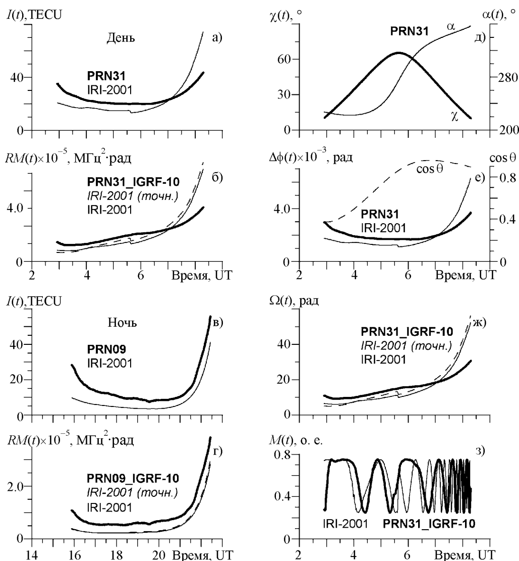
Рис. 6. Передаточные характеристики ионосферы в районе радиотелескопа MIRA для магнитной бури 30 октября 2003 г.
