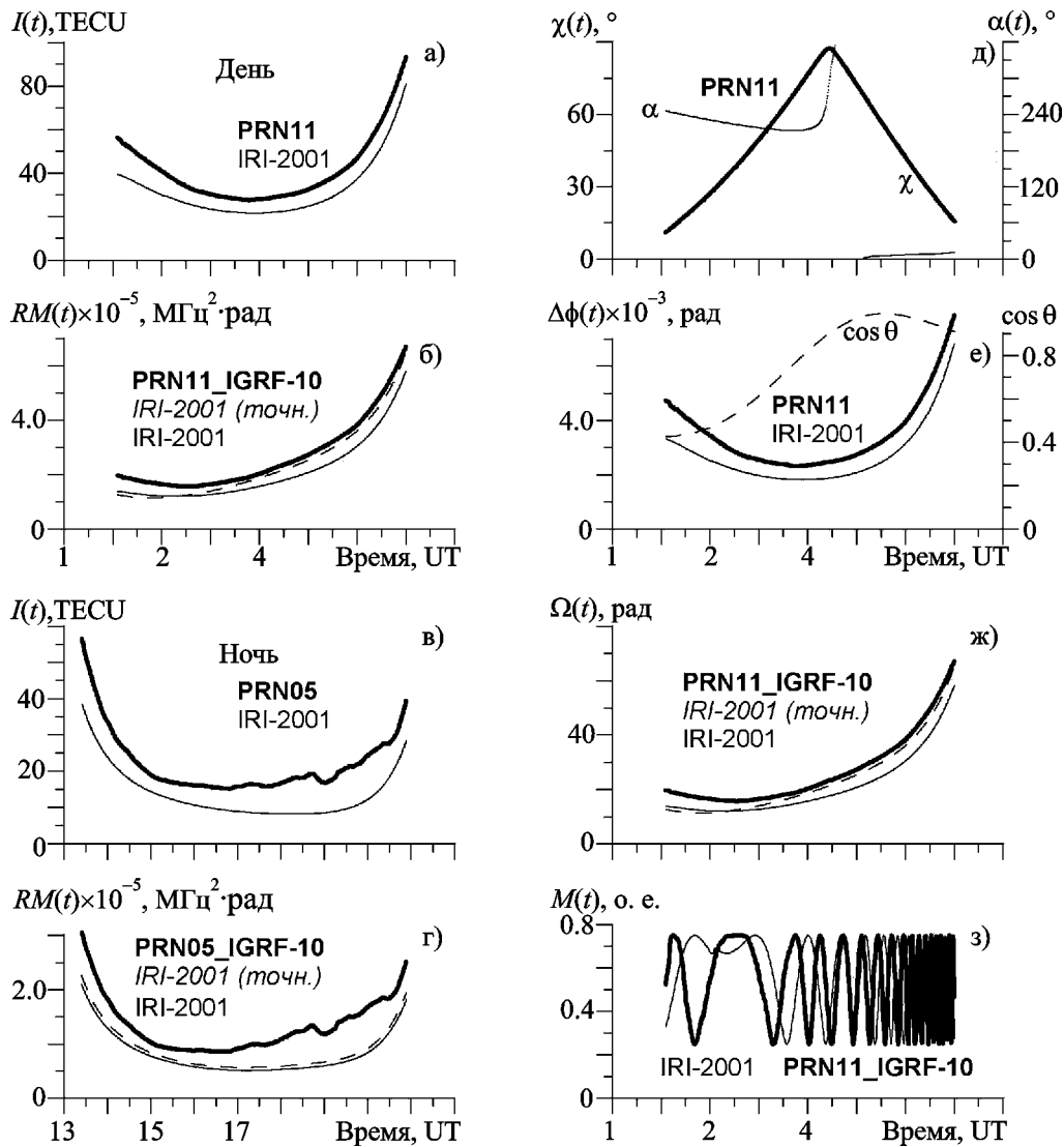
Рис. 5. Передаточные характеристики ионосферы в районе радиотелескопа MIRA для магнитоспокойного дня 4 декабря 2004 г.
