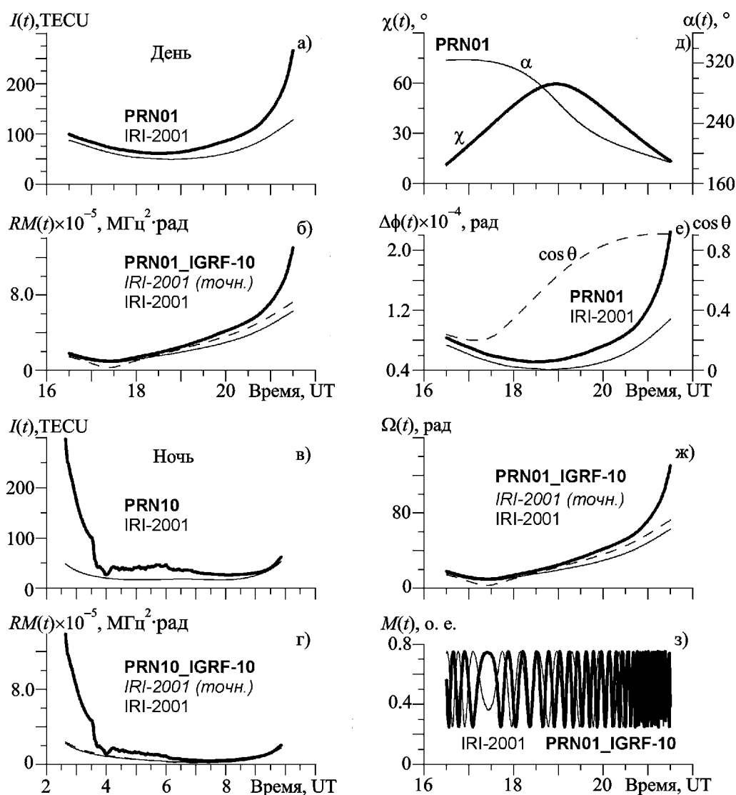
Рис. 8. Передаточные характеристики ионосферы в районе радиотелескопа Arecibo для магнитной бури 30 октября 2003 г.
