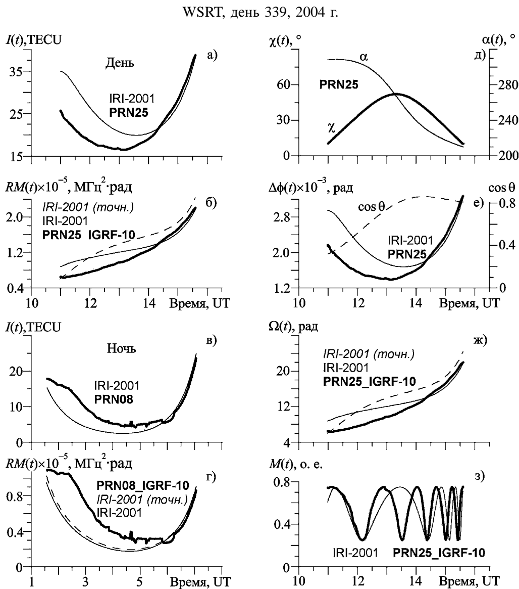
Рис. 3. Передаточные характеристики ионосферы в районе радиотелескопа LOFAR для магнитоспокойного дня 4 декабря 2004 г.: а), в) – наклонное ПЭС I(t) (жирные кривые – данные GPS станции WSRT, тонкие кривые – модель IRI-2001); б), г) – мера вращения RM(t) (жирные кривые – экспериментальные данные, тонкие кривые – приближенный расчет IRI-2001, пунктирные кривые – точный расчет IRI-2001); д) – азимут \alpha(t) и угол места \chi(t) луча зрения от станции WSRT на ИСЗ PRN25 (тонкая и жирная линии соответственно); е), ж), з) – рассчитанные для частоты 100 МГц фазовое запаздывание \Delta\phi(t) , угол поворота плоскости поляризации \Omega(t) и модулирующая функция ФАМ M(t) соответственно (обозначения те же, что на панелях б) и г), пунктирная кривая на панели е) – зависимость \cos\theta(t) ). На панелях отмечены номера спутников GPS (PRN)
