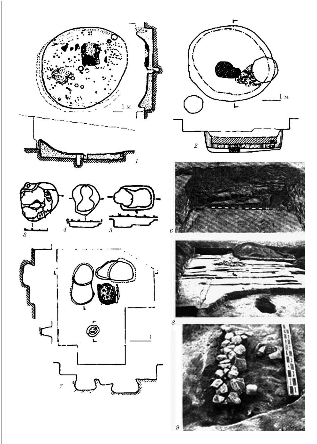
Рис. 2. 1, 2 — планы и разрезы землянок (Немировское городище); 3—5 — планы полуземлянок (поселение Вишенка II); 6 — разрез землянки (Гясминское городище); 7 — остатки наземного жилища (Немировское городище); 8 — остатки наземного жилища (поселение Непорогово); 9 — остатки каменного фундамента жилого сооружения (поселение Непорогово)
