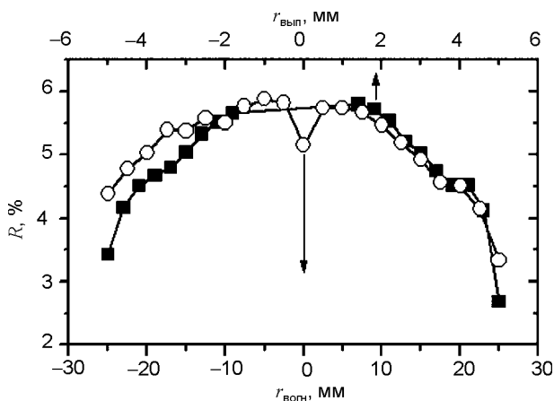
Рис. 8. Распределение коэффициентов отражения вдоль радиуса выпуклого (■) и вогнутого (○) зеркал в области “углеродного окна”.
