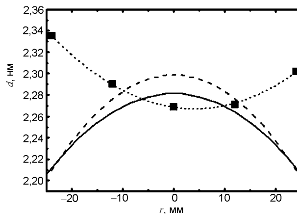
Рис. 4. Расчетные (—, ----) зависимости периода покрытия на вогнутом зеркале для двух выпуклых зеркал, приведенных на рис. 2 (○, □, соответственно) и экспериментально полученное (·-■·) распределение периода до применения градирующих период методик.
