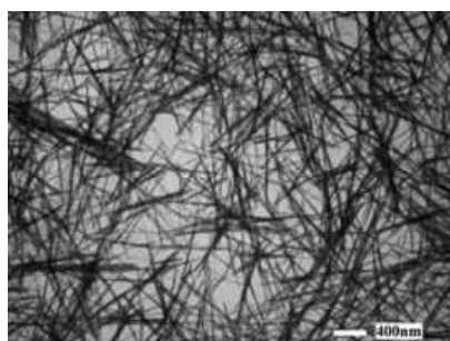
Рис. 5. Морфология нанонитей Gd_{0.97}Eu_{0.03}PO_4 , полученных осаждением из водных растворов с использованием ультразвука.
