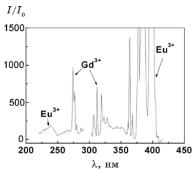
Рис. 3. Спектр возбуждения Gd_{0.44}Y_{0.54}Eu_{0.02}PO_4 .
