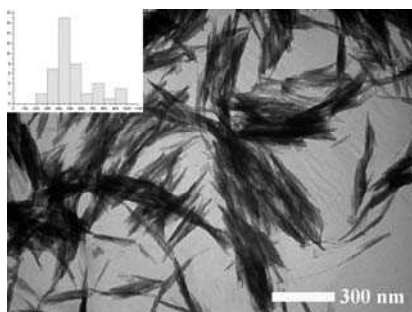
Рис. 6. ПЭМ-изображение Gd_{0.97}Eu_{0.03}PO_4 , полученного в микроэмульсиях в течение 5 часов и T = 21^\circ C .
