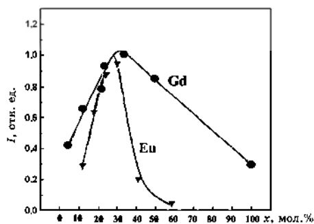
Рис. 4. Нормированный квантовый выход люминесценции в фосфорах Y_{1-x-y}Gd_xEu_yPO_4 .
