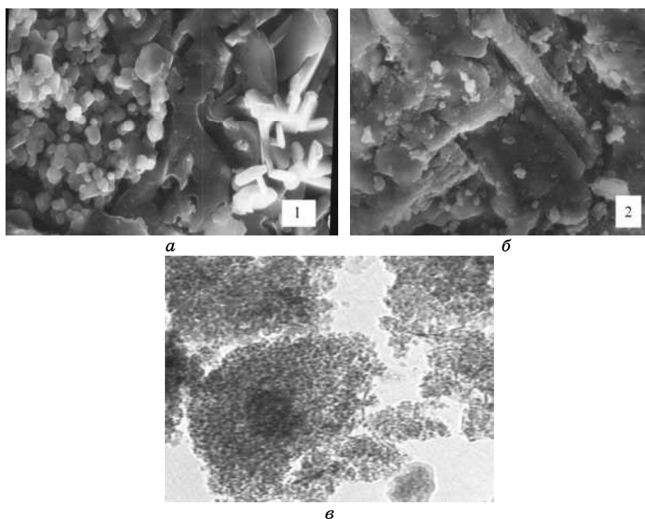
Рис. 2. Микроструктура кордиеритовой матрицы (а) и композита с волокнистым наполнителем (б), отожженных при 1200°C, ув. 5000; (в) — фрагмент волокна, состоящий из нанозерен оксида алюминия, ув. 100000.
