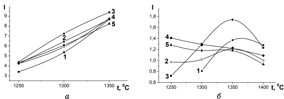
Рис. 1. Изменение интегральных интенсивностей рефлексов кристаллических фаз: кордиерита (а) и алюмомагниевого шпинели (б) в поликомпонентной керамической матрице (1) и композитах с наполнителем \text{Al}_2\text{O}_3 : 2 — 5 масс.%, 3 — 10 масс.%, 4 — 15 масс.% и 5 — 20 масс.%.
