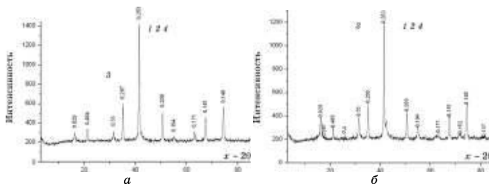
Рис. 4. Рентгенофазовый анализ полученных наноразмерных железо-кислородных структур верхний слой (а) и нижний слой (б) на железном диске без влияния магнитного поля. Фазовый состав: 1 — \gamma\text{-Fe}_2\text{O}_3 , 2 — \text{Fe}_3\text{O}_4 , 3 — \gamma\text{-FeOOH} , 4 — \text{Fe}(\text{OH})_3
