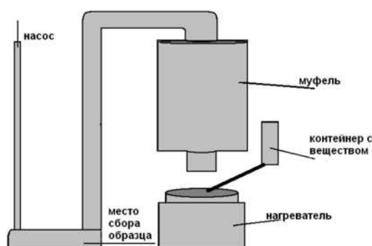
Рис. 2. Схема установки для получения TiO_2 .
