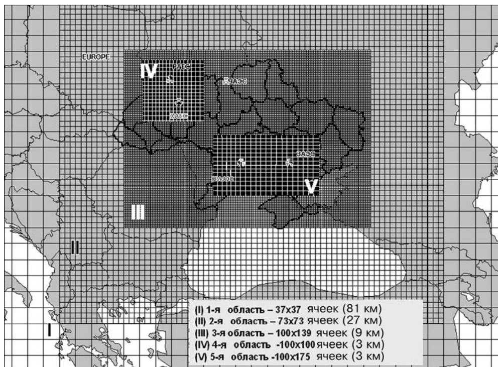
Рис. 2. Области счета.
