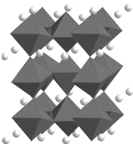
Рис. 6. Схема структуры перовскита LCMO с выделенными октаэдрами MnO 6 . Кружки отображают катионы La 3+ и Ca 2+ (масштабы не соблюдены)
