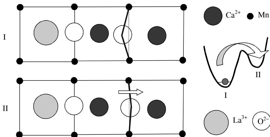
Рис. 7. Варианты искажения связей Mn–O–Mn при соседстве катионов одного размера: I – соответствует локальному минимуму энергии, II – метастабильному состоянию
