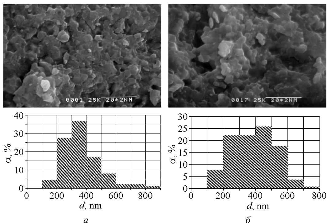
Рис. 2. Поверхности изломов образцов посредством изгиба ( a ) и механического ударного разрушения ( b ) и характеризующие их гистограммы: a – \langle d \rangle = 366 \text{ nm} , b – \langle d \rangle = 387 \text{ nm}
