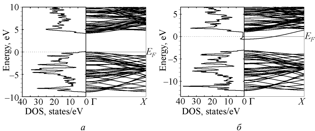
Рис. 1. Плотность электронных состояний и зонная структура бор-азотной НТ типа «зигзаг» (12, 0): а – идеальной, б – заполненной калием
