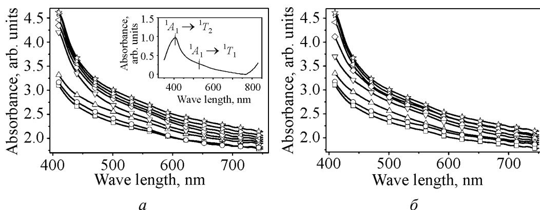
Рис. 1. Спектры поглощения \text{Fe(3-Fru)}_2\text{Ni(CN)}_4 при дискретном повышении (а) и понижении (б) давления, GPa: а: \square - 10^{-4} , \circ - 0.247 , \triangle - 0.333 , \nabla - 0.427 , \diamond - 0.488 , \triangleleft - 0.614 , \triangleright - 0.775 , \star - 0.931 ; б: \square - 10^{-4} , \circ - 0.123 , \triangle - 0.225 , \nabla - 0.304 , \diamond - 0.393 , \triangleleft - 0.505 , \triangleright - 0.727 , \star - 0.931 . На вставке изображен спектр пропускания соединения при давлении 0.931 GPa во всей области спектральной чувствительности экспериментальной установки от 330 до 840 nm
