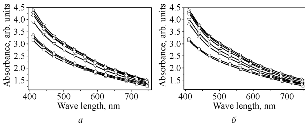
Рис. 2. Спектры поглощения \text{Fe(3-Fru)}_2\text{Pt(CN)}_4 при дискретном повышении (а) и понижении (б) давления, GPa: а: \square - 10^{-4} , \circ - 0.130 , \triangle - 0.242 , \nabla - 0.353 , \diamond - 0.477 , \triangleleft - 0.719 , \triangleright - 0.878 ; б: \square - 10^{-4} , \circ - 0.177 , \triangle - 0.261 , \nabla - 0.302 , \diamond - 0.366 , \triangleleft - 0.700 , \triangleright - 0.878
