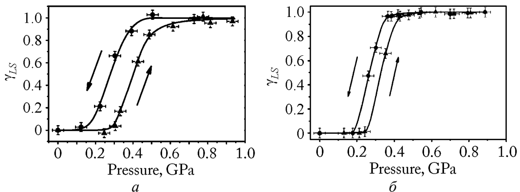
Рис. 3. Зависимости доли высокоспиновой фазы от давления соединений: a – Fe(3-Fpy)_2Ni(CN)_4 , б – Fe(3-Fpy)_2Pt(CN)_4 . Для наглядности переходов сплошные линии проведены от руки
