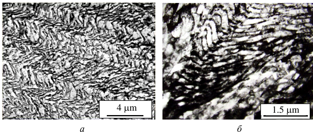
Рис. 12. Визуализация картин течения при наличии выделений вторых фаз: а – Ti–5Mo–5V–5Al, гидроэкструзия, \varepsilon = 30\% ; б – Fe–0.3% C, деформация сдвигом, e = 4
