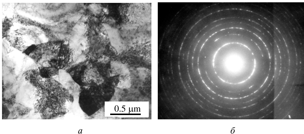
Рис. 14. Сплав Ti–40Nb после гидроэкструзии ( \epsilon = 34\% ): а – экстинкционные контуры и фрагменты в структуре сплава; б – микродифракция
