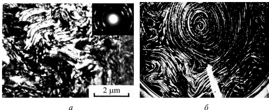
Рис. 2. Структура сплава Fe–17Ni–10W–10Co–1Mo–1Ti после гидроэкструзии 87% ( a ) и ее подобие с конвекцией жидкости (с алюминиевыми частицами) во вращающемся цилиндре, нагретом по внешней поверхности и охлажденном в центре ( б ) [22]
