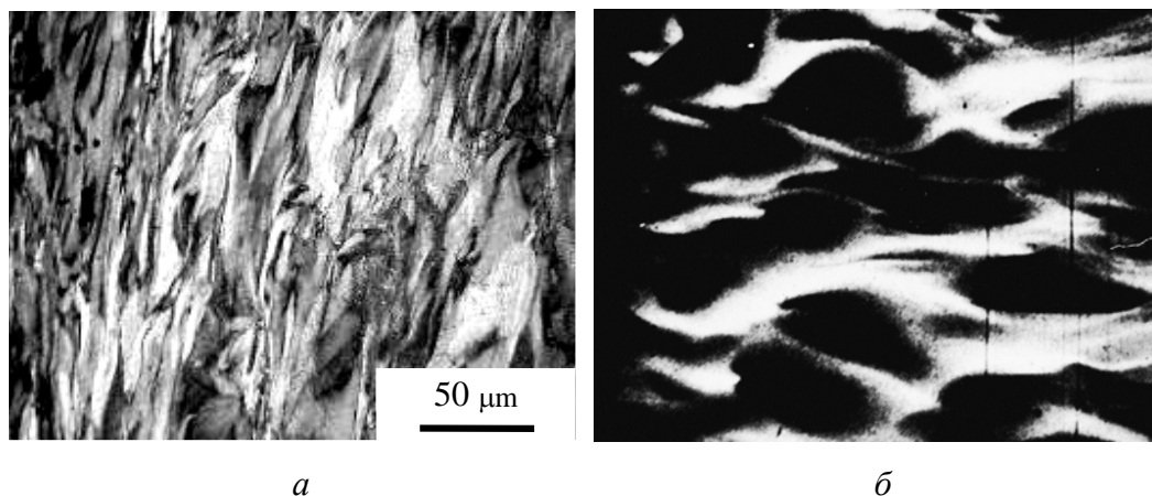
Рис. 1. Структура титанового сплава Ti–5Mo–5V–5Al на периферии образца после 1 цикла винтовой экструзии при 300°C ( a ) и ее аналогия со структурой подслоя турбулентного пограничного слоя ( б ) [22]. Визуализация осуществлена с помощью алюминиевых частиц в глицерине
