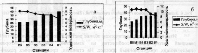
Рис. 7. Изменение удельной поверхности популяций Phyllophora crispata (Huds.) P.S. Dixon (а) и Ph. truncata (Pall.) Zinova (б) с глубиной.
