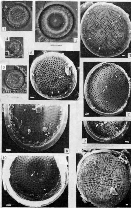
Табл. I. Concentrodiscus subabnormis Khursevich & Fedenya sp. nov.: 1 – общий вид, СМ; 3, 6, 11 – наружная поверхность створки с неотчетливыми пучками ареол на лицевой части и краевым кольцом коротких трубок выростов с опорами на загибе створки (стрелки, 3, 6), СЭМ; 7, 10 – фрагмент внутренней поверхности створки с одним двугубым выростом близ центра (стрелки), СЭМ; 8, 9 – фрагмент внутренней поверхности створки с одним двугубым выростом на границе лицевой части створки и загиба (стрелки) и краевым кольцом выростов с 4 сателлитными порами на загибе створки, СЭМ. Concentrodiscus indigenus Khursevich & Fedenya: 2 – общий вид, СМ. Concentrodiscus proteus Khursevich & Fedenya sp. nov.: 4, 5 – общий вид, СМ. Масштаб: 1, 2, 4, 5 – 10 мкм, 3, 6 – 11 – 1 мкм.
