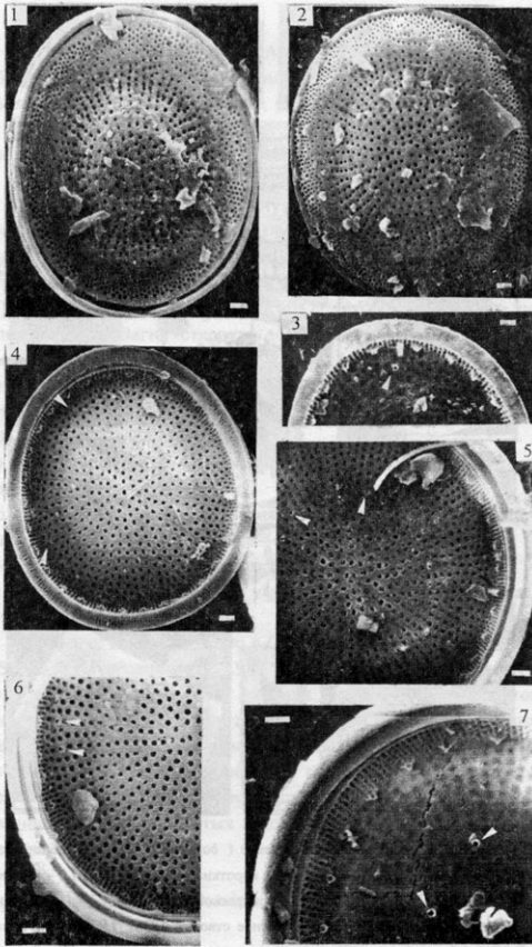
Табл. III. Concentrodiscus indigenus Khursevich & Fedena: 1, 2 – наружная поверхность створки с отчетливой концентрической волнистостью, СЭМ; 3, 4, 6 – фрагмент внутренней поверхности створки с двугубым выростом на загибе створки и кольцом выростов с 4 сателлитными порами в прикраевой зоне лицевой части (стрелки), СЭМ; 5, 7 – фрагмент внутренней поверхности створки с двугубым выростом на загибе створки (черная стрелка), 5) и кольцом выростов с опорами в центральной зоне створки (белые стрелки), СЭМ. Масштаб: 1-7 – 1 мкм.
