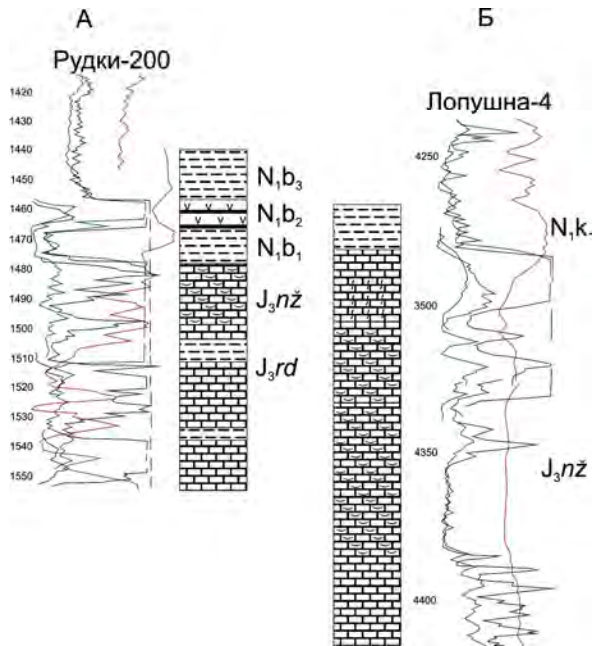
Рис. 1. Типові розрізи верхньої юри зі свердловин Рудки-200 (А) і Лопушня-4 (Б) А: біогермний вапняк оксфорд, перекритий регіональною покришкою гіпсо-ангідритового горизонту бадену; Б: біогермний вапняк титону, перекритий локальною покришкою щільного нижньокрейдового вапняку
