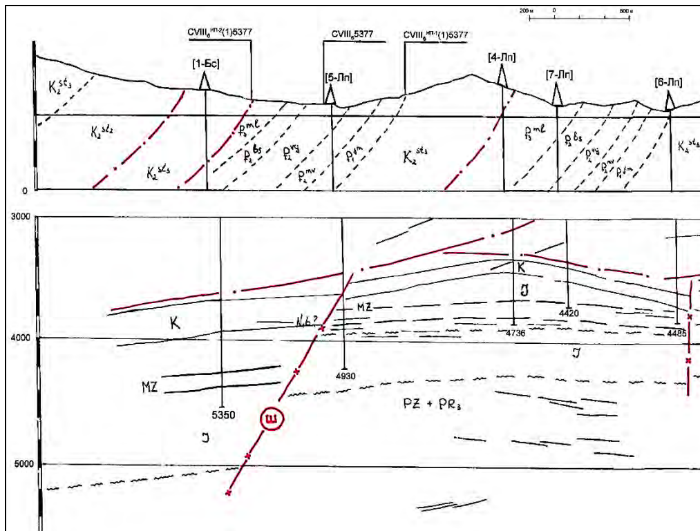
Рис. 2. Фрагмент сейсмогеологічного профілю, Лопушнянська площа (11 6 5377)
