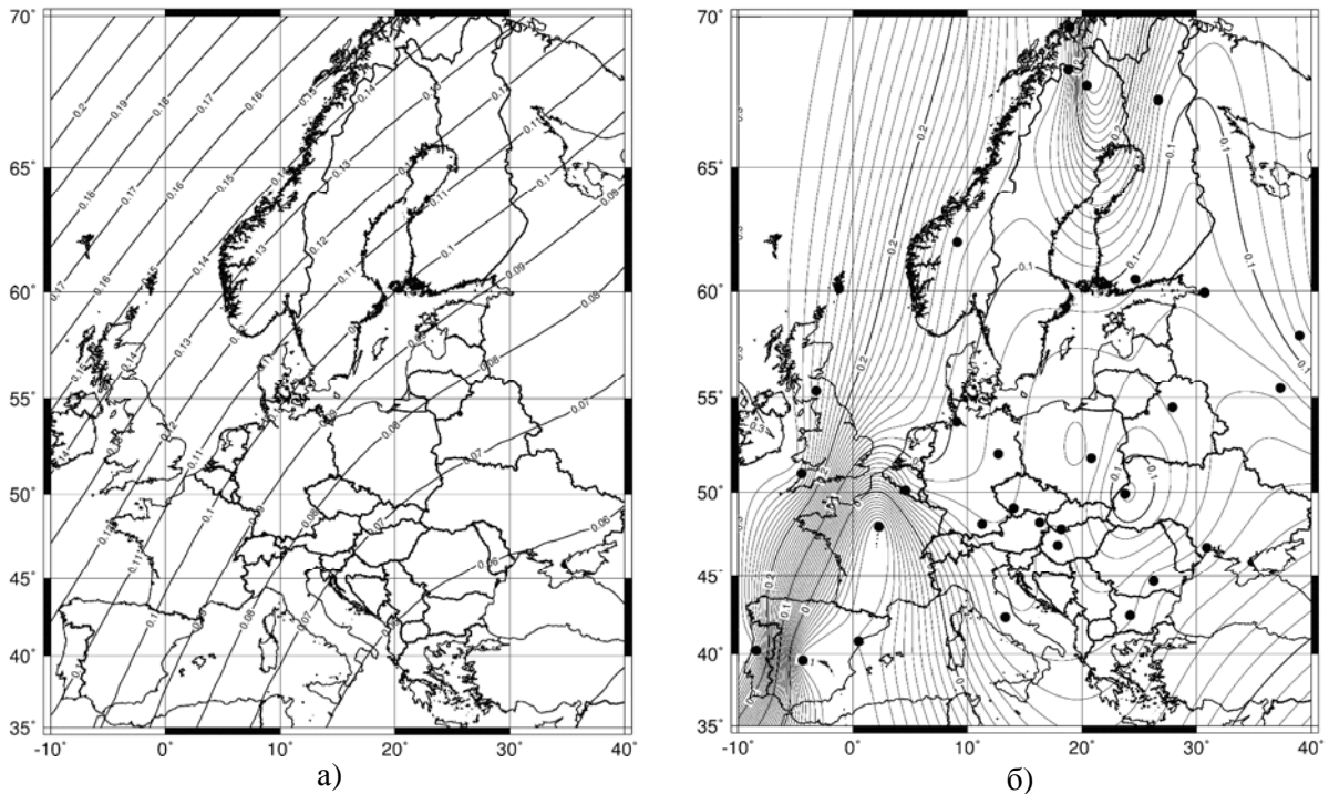
Рис. 10. Структура вікової варіації D-компоненти геомагнітного поля на території Європи впродовж 2000–2005 рр. а) – розрахунки за IGRF; б) – за даними МО; значення ізоліній у \text{nT}/\text{рік}
