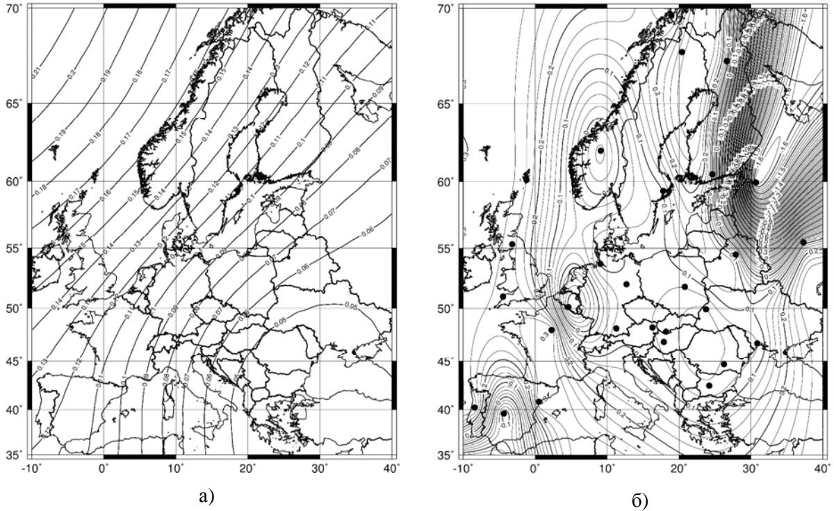
Рис. 9. Структура вікової варіації D-компоненти геомагнітного поля на території Європи впродовж 1995–2000 рр.: а) – розрахунки за IGRF; б) – за даними МО; значення ізоліній у ^{\circ}/\text{рік}
