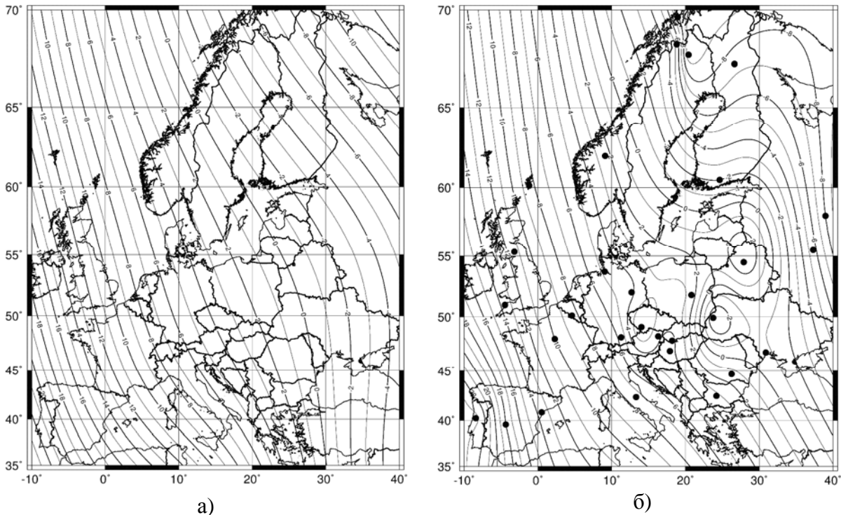
Рис. 4. Структура вікової варіації X-компоненти геомагнітного поля на території Європи впродовж 2000–2005 рр.: а) – розрахунки за IGRF; б) – за даними МО; значення ізоліній в нТл/рік
