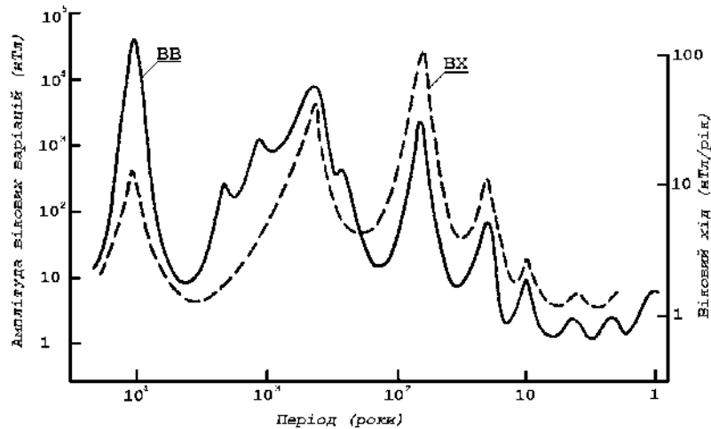
Рис. 1. Спектр вікових варіацій геомагнітного поля (BB – вікова варіація, BX – віковий хід)
