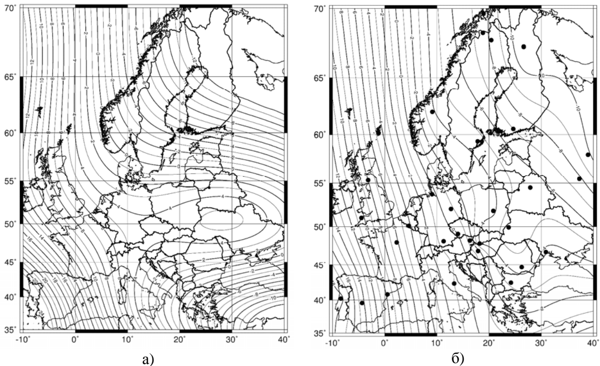
Рис. 3. Структура вікової варіації X-компоненти геомагнітного поля на території Європи впродовж 1995–2000 рр.: а) – розрахунки за IGRF; б) – за даними МО; значення ізоліній в нТл/рік
