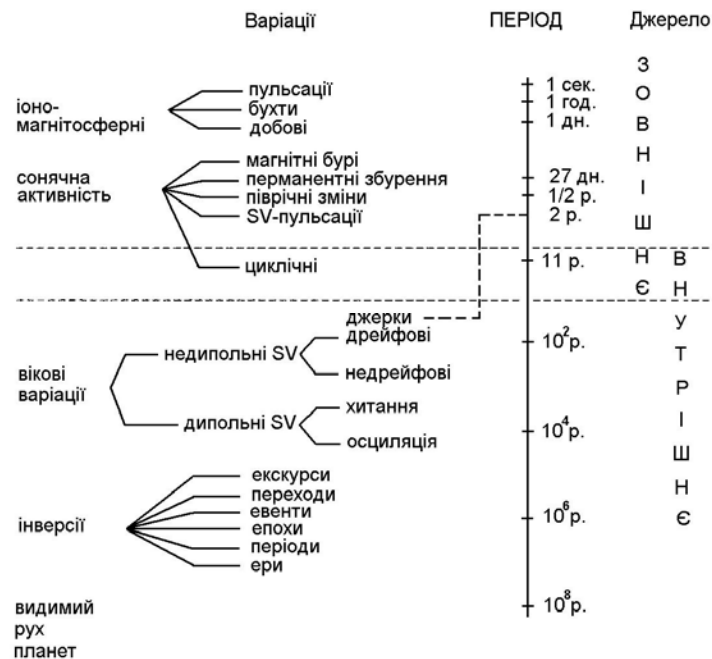
Рис. 2. Схема спектрального розподілу варіацій геомагнітного поля та локалізація їх джерел
