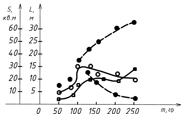
Рис. 1. Залежність дальності руху газодисперсного конгломерата L та площі його ефективного впливу S від величини розпилювального заряду — m .
