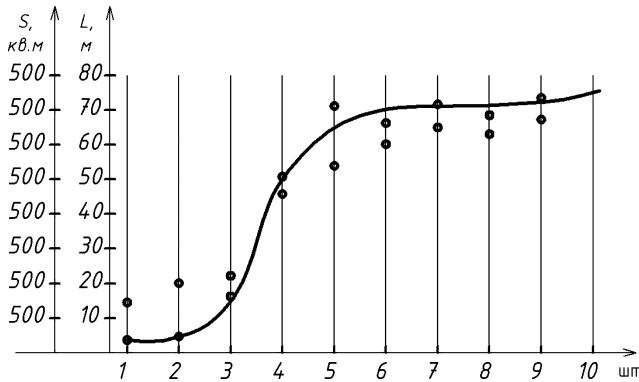
Рис. 3. Залежність дальності распылення L і його площі S від кількості стволів N учасуючих в залпе.
