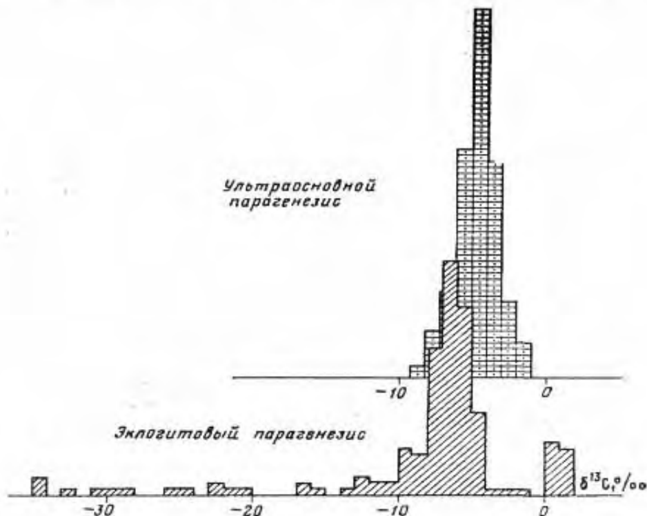
Рис. 11. Изотопный состав углерода алмазов ультраосновного и эклогитового парагенезисов по Э. М. Галимову [6].
