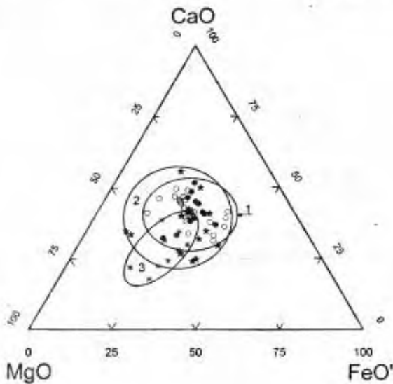
Рис. 8. Диаграмма CaO–MgO–FeO общ : 1 — поле базальтов срединно-океанических хребтов, построенное по данным [34] и габбро океанической коры [13]; 2 — поле эклогитов Южной Африки по данным [8]; 3 — поле эклогитов Якутии по данным [10].
