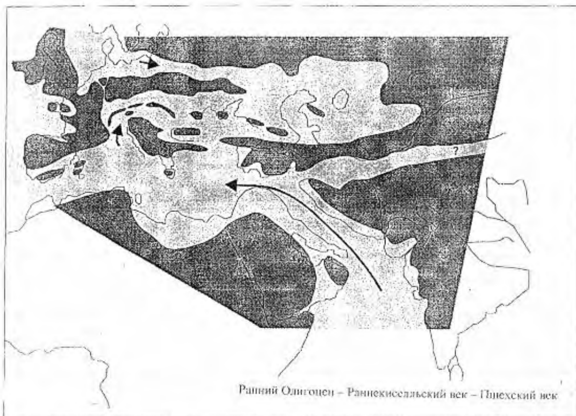
Рис. 5. Зарождение морского бассейна Паратетис. Вследствие тектонической активности по альпийскому фронту и коллизии Индии с Евразией возникли внутриконтинентальное море Паратетис, а к югу от орогена – Средиземное море. Вследствие нарастания континентализации и произошло закрытие Тургайского пролива. По вновь образованным системам проливов атлантическая вода из Северного моря поступала в Паратетис [42].
