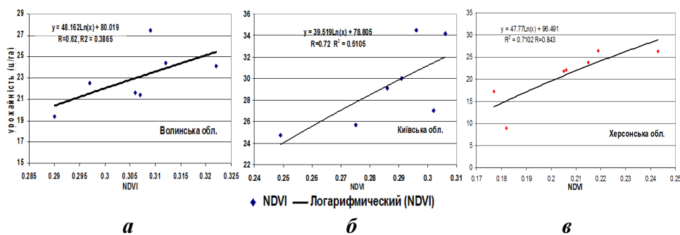
Р и с . 1 . Кореляційна залежність між урожайністю зернових культур і показником NDVI : Полісся (а), Лісостеп (б), Степ (в).
