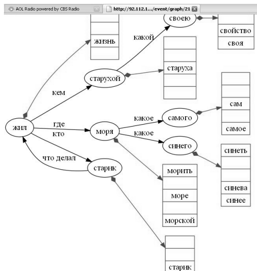
Рис. 4. Режим графической интерпретации связей синтагмы
