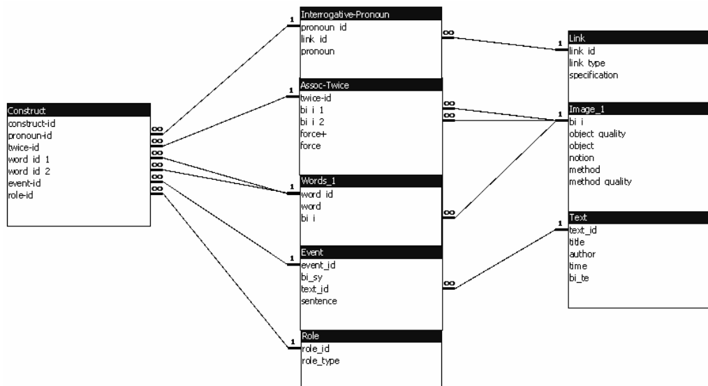
Рис. 1. Схема данных тезауруса образов
