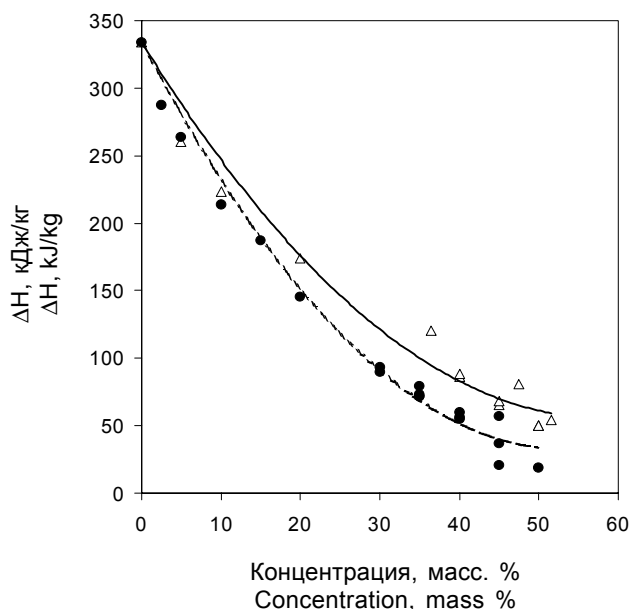
Рис. 7. Зависимость теплоты плавления водных растворов глицерина (●) и 1,2-ПД (Δ) от их массовых концентраций.
