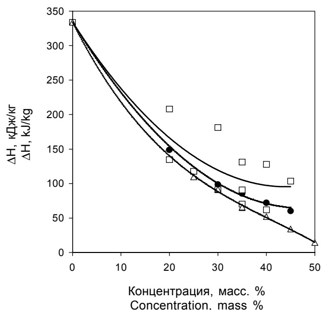
Рис. 8. Зависимость теплоты плавления водных растворов бутандиолов от их массовых концентраций: ● – 1,3-БД; □ – 2,3-БД; Δ – Levo-2,3-БД.
