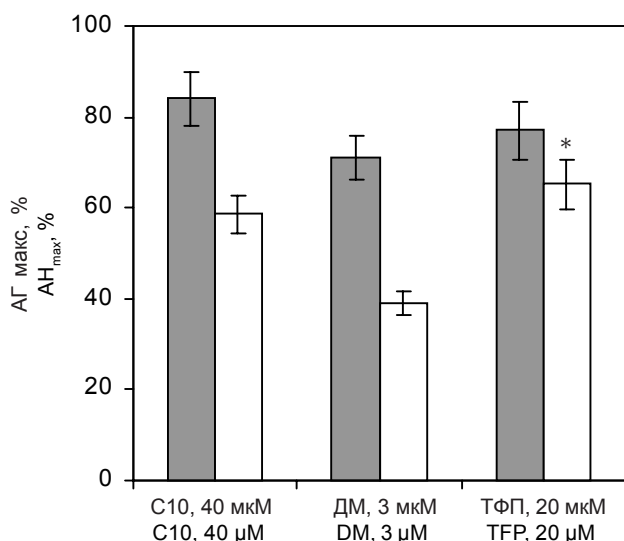
Рис. 2. Антигемолитическая активность амфифильных веществ в условиях гипертонического гемолиза (4,0 М NaCl) эритроцитов лошади при температуре 37°C: ■ – контроль; □ – клетки, предварительно инкубированные при 49°C; * – различия достоверны по сравнению с контролем, P < 0,05 . На оси представлены эффективные концентрации используемых амфифильных соединений.
