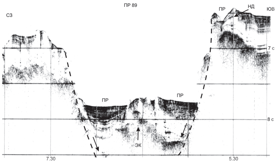
Рис. 7. Фрагмент профиля НСП 89 через рифтограбен (раздвиг), заполненный контрастными неоген-раннечетвертичными турбидитами (зона разлома Хоккайдо [14]). ЭК – экструзивный купол, ПР – подводное русло, НД – намывная дамба (НИС “Проф. Гагаринский”-1989). Координаты ПК 5.30 (44° 42,50 с.ш., 157° 22,62 в.д.) и ПК 7.30 (44° 32,57 с.ш., 157° 44,63 в.д.)
