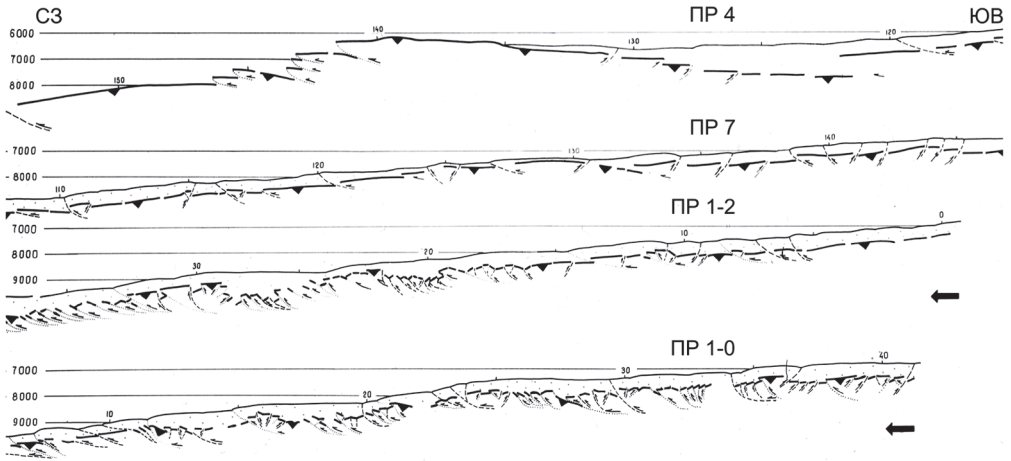
Рис. 3. Глубинные разрезы НСП 4,7 и МОГТ 1-2,1-0 по внешнему склону южной части Курильского жёлоба (м-б 1:1) [13]. Чешуйчатые надвижки смещают дно и кровлю слоя 2
