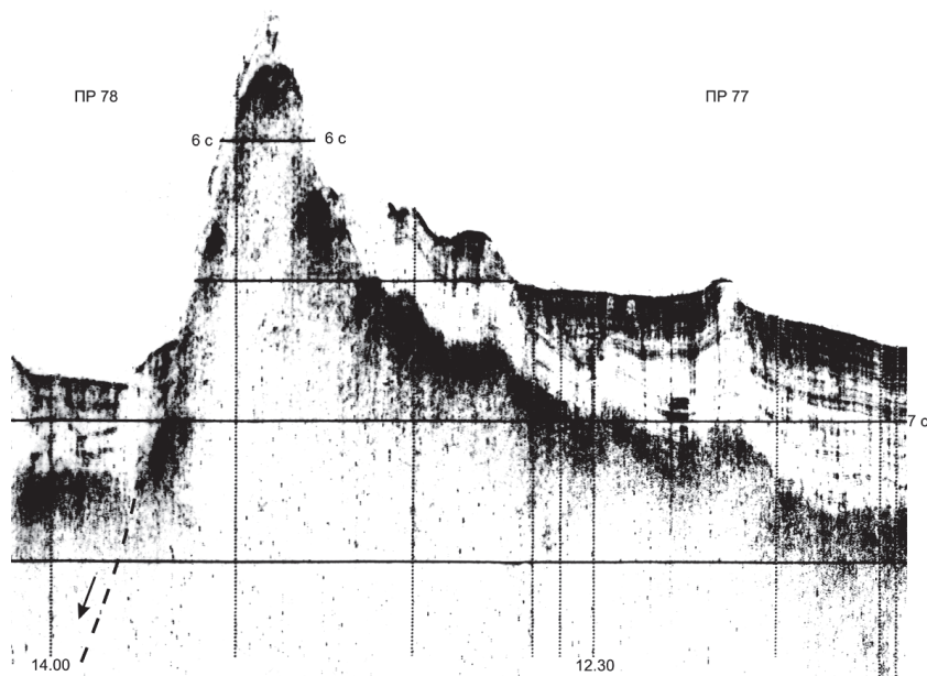
Рис. 8. Профили НСП 77, 78 через южный борт рифтограбена (раздви́г) с экстрезивной одиночной горой в зоне разлома Хоккайдо (НИС “Проф. Гагаринский”-1989). Координаты ПК 12.30 (45° 06,14 с.ш., 157° 01,98 в.д.) и ПК 14.00 (45° 12,29 с.ш., 157° 17,90 в.д.)
