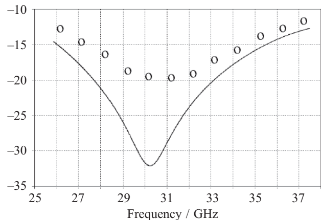
Рис. 4. Развязка между выходными волноводами (дБ)
