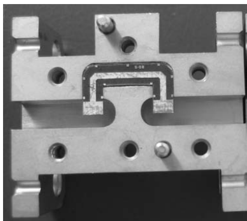
Рис. 2. Общий вид исследуемой конструкции ВМП
