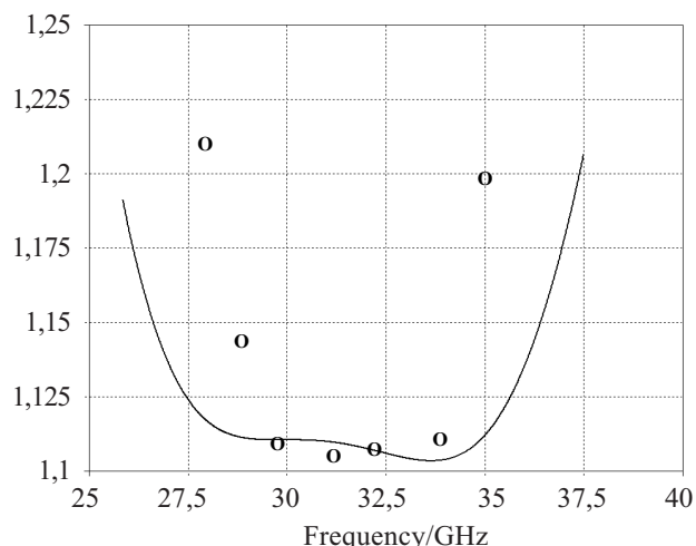
Рис. 3. Расчетные и экспериментальные (o) значения КСВН ВМП
