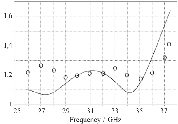
Рис. 2. КСВН входного волновода
