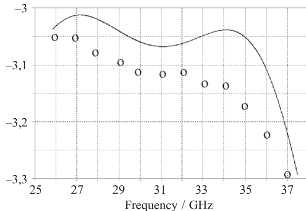
Рис. 3. Потери передачи из входного волновода в выходной (дБ)
