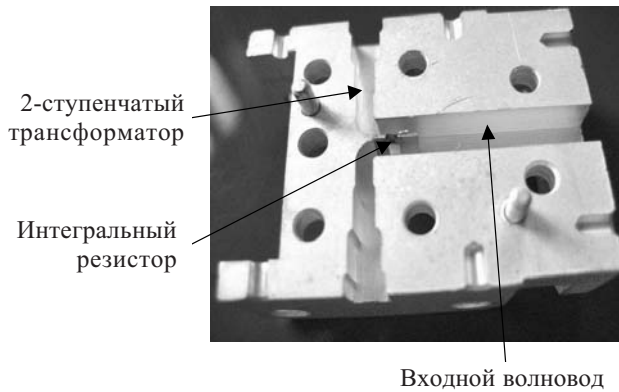
Рис. 1. E -плоскостной делитель со снятой верхней частью
