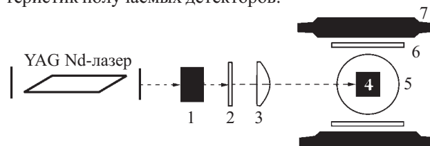
Рис. 1. Схема установки для лазерной абляции и фотостимулированной пассивации боковой поверхности образцов Cd_{1-x}Zn_xTe :
