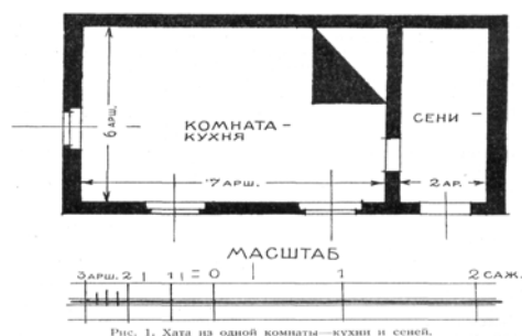
Рис. 1. Хата із однієї кімнати—кухні і сеней.
