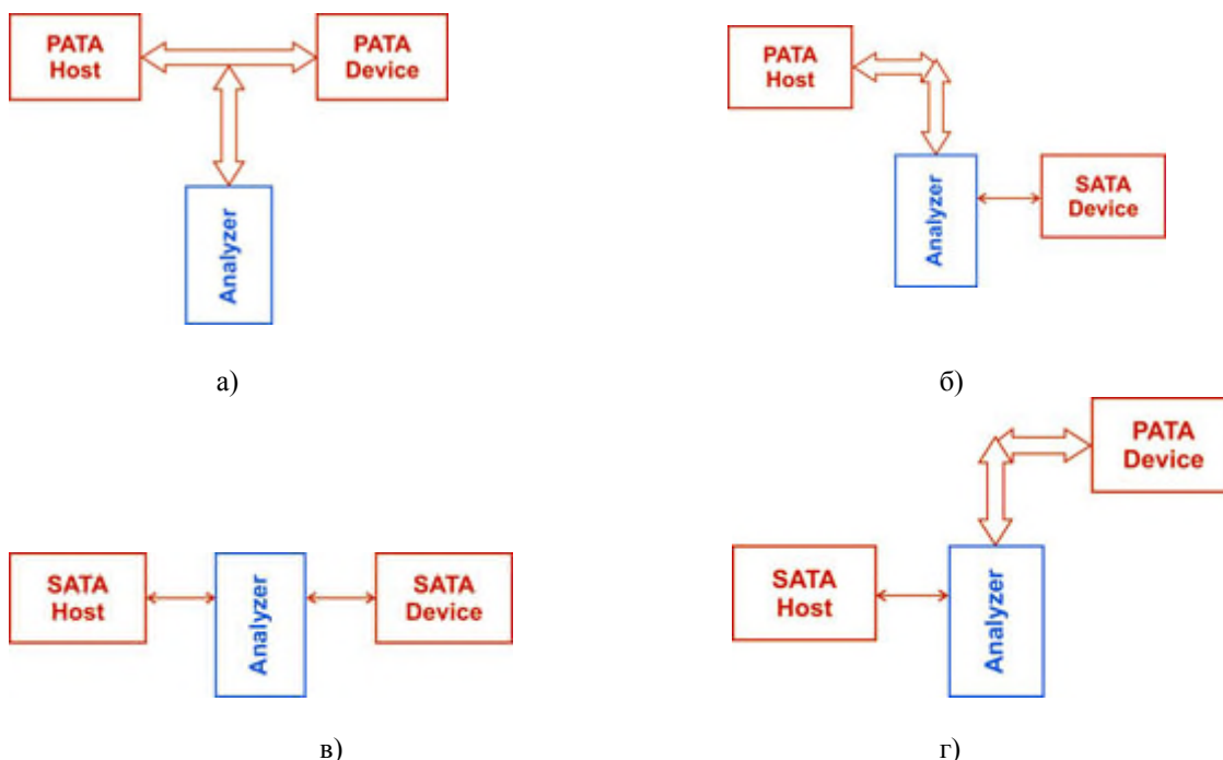
Рис. 4. Схемы подключения анализатора EPOS ATA Analyzer: а) PATA-хост → PATA-устройство; б) PATA-хост → SATA-устройство; в) SATA-хост → SATA-устройство; г) SATA-хост → PATA-устройство
