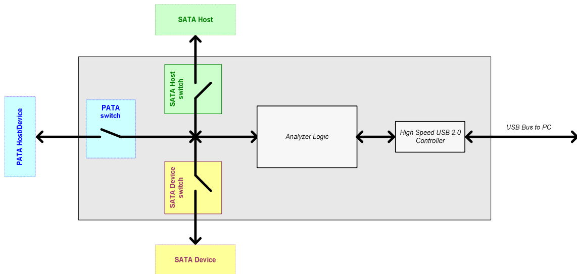
Рис. 3. Структурная схема анализатора протокола EPOS ATA Analyzer
