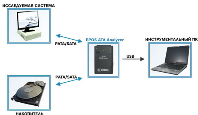
Рис. 1. Типовая схема подключения анализатора протокола EPOS ATA Analyzer
