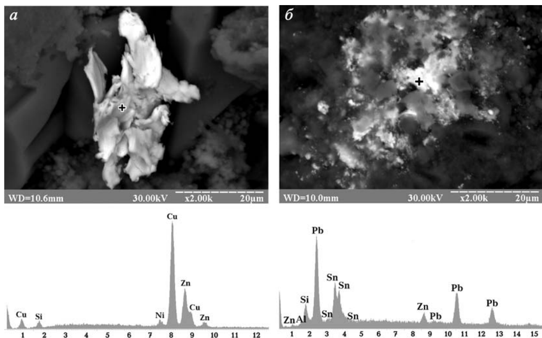
Рис. 22. Самородная цинкистая медь (природная латунь) с примесью никеля (а) и природный сплав свинца и олова (с примесью цинка) (б) в песчаном коллекторе-метасоматите (нефтяное месторождение Субботина, скв. 1, 2490,2–2495,8 м)
