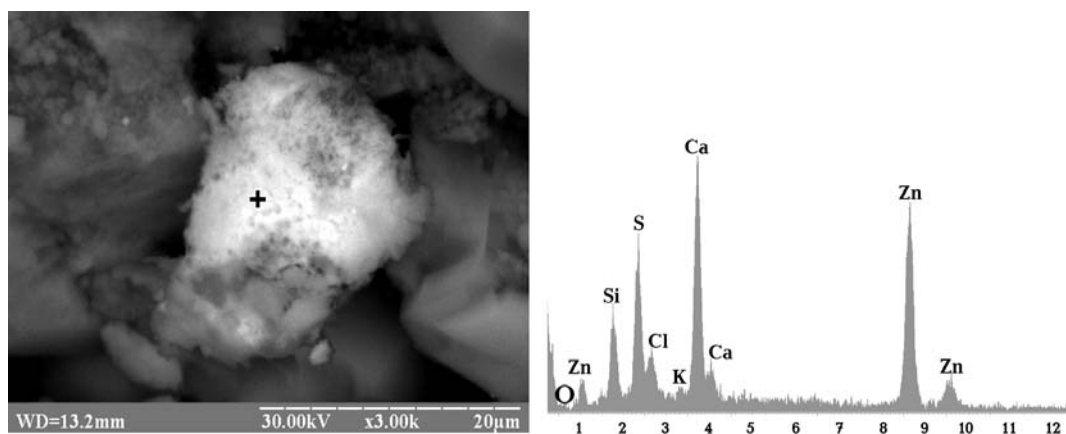
Рис. 23 Зернисто-волокнистый агрегат самородного цинка, сфалерита и цинкита (?) в песчаном коллекторе-метасоматите (нефтяное месторождение Субботина, скв. 1, 2490,2–2495,8 м)
