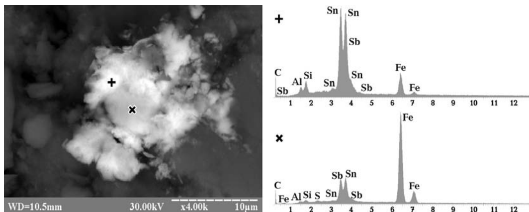
Рис. 12. Агрегат самородных металлов: железо, олово, сурьма (грязевый вулкан Джау-Тепе, Керченский п-ов), карбонатная корка (фумарольное образование)
