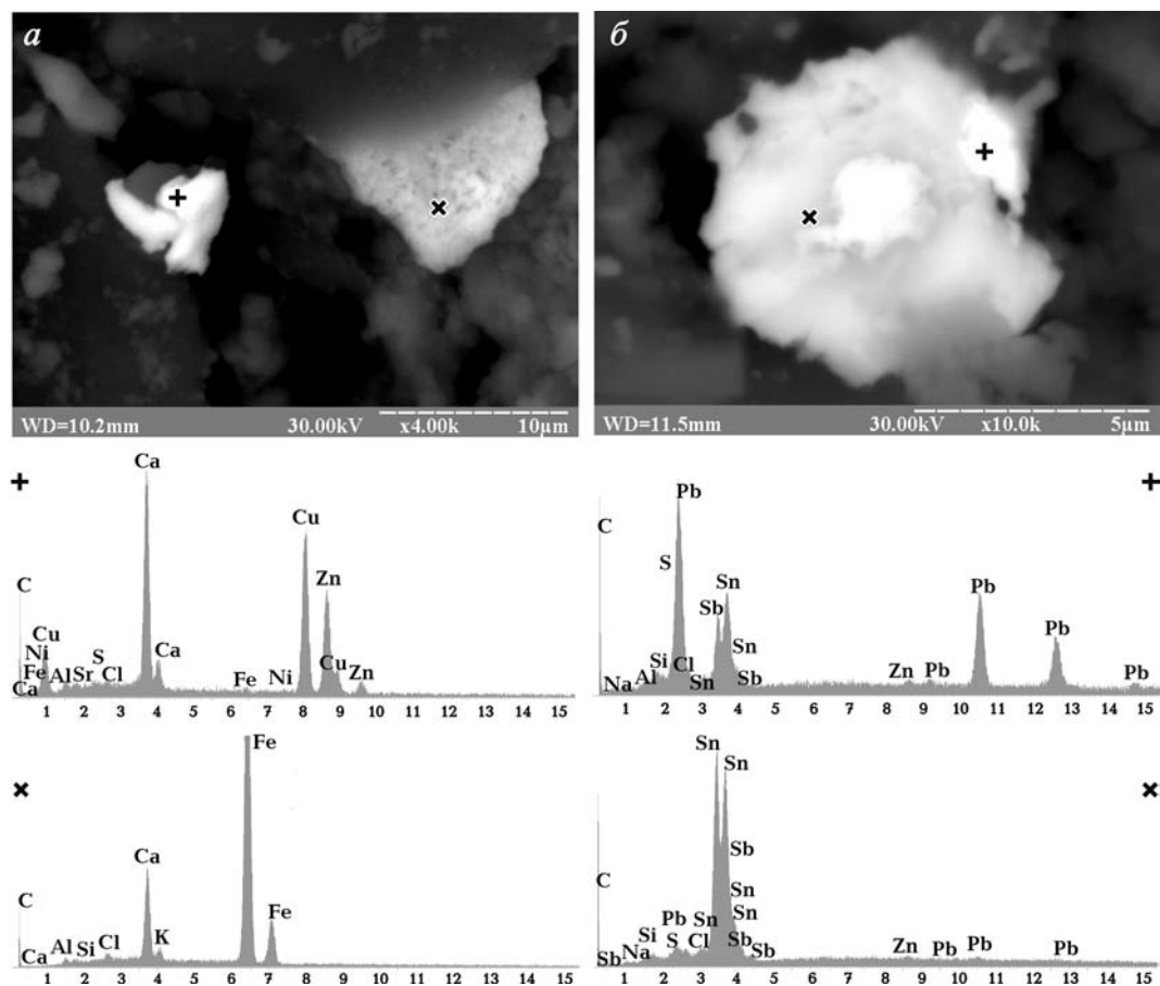
Рис. 8. Сплав меди с цинком и никелем (природная латунь – бронза) (а) и агрегат самородного свинца и сплава олова с сурьмой (б) в гераклите
