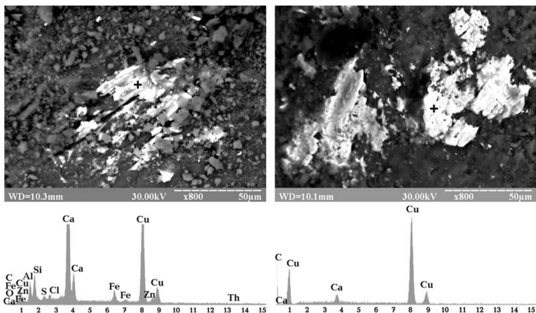
Рис. 6. Самородная медь гераклите
