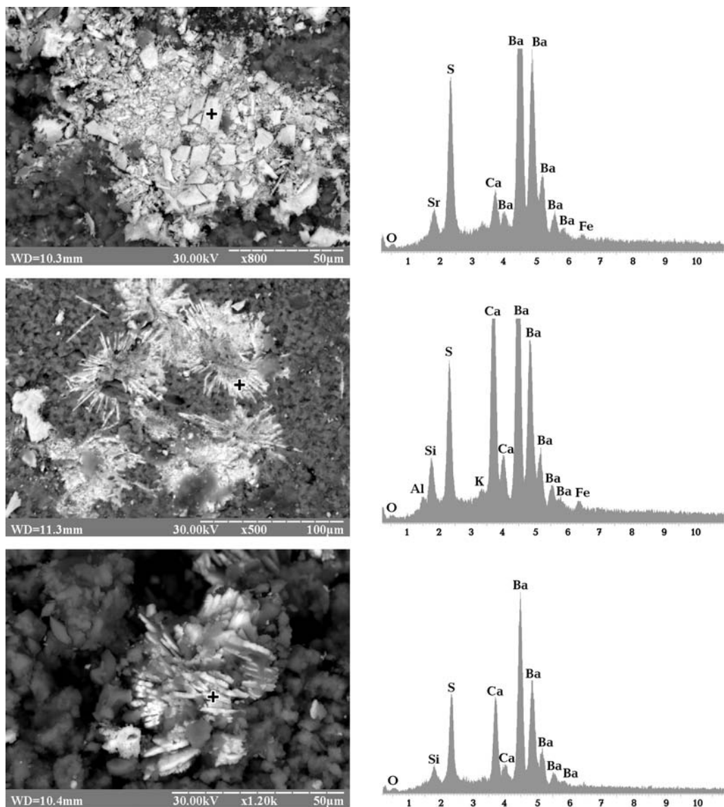
Рис. 14. Барит-карбонатная корка (твердая часть) (грязевый вулкан Двуреченский, прогиб Сорокина, Черное море)
