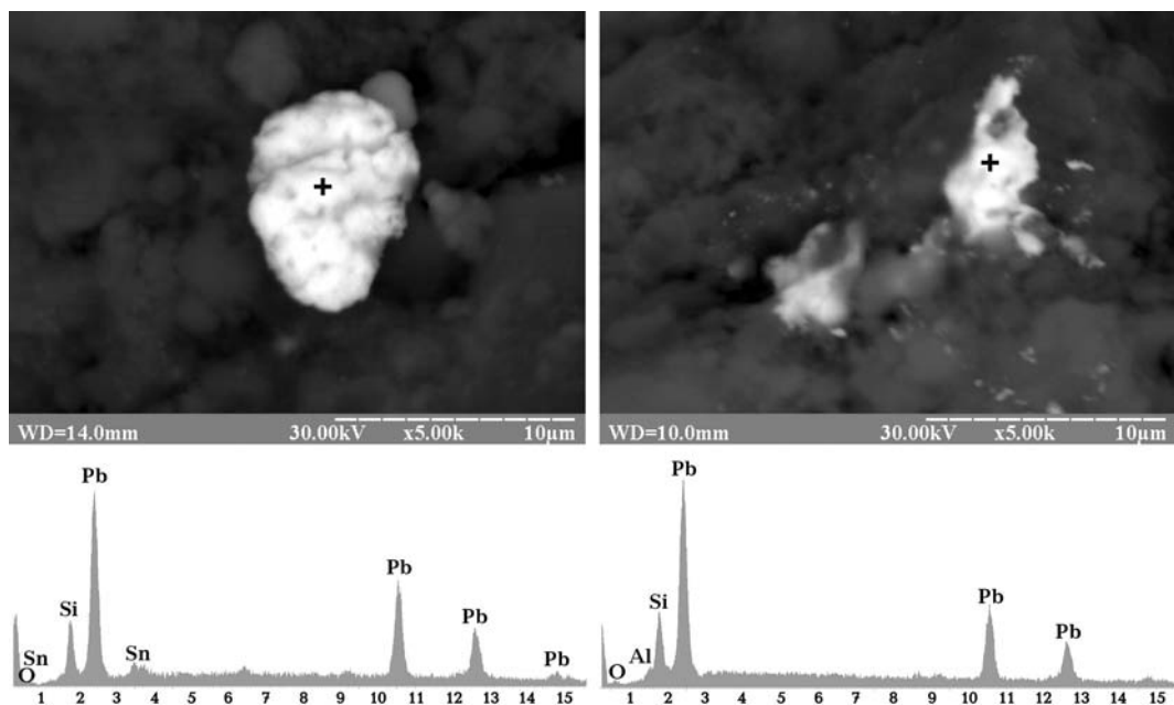
Рис. 21. Самородный свинец (относительно чистый и с примесью олова) в песчаном коллекторе-метасоматите (нефтяное месторождение Субботина, скв. 1, 2490,2–2495,8 м)
