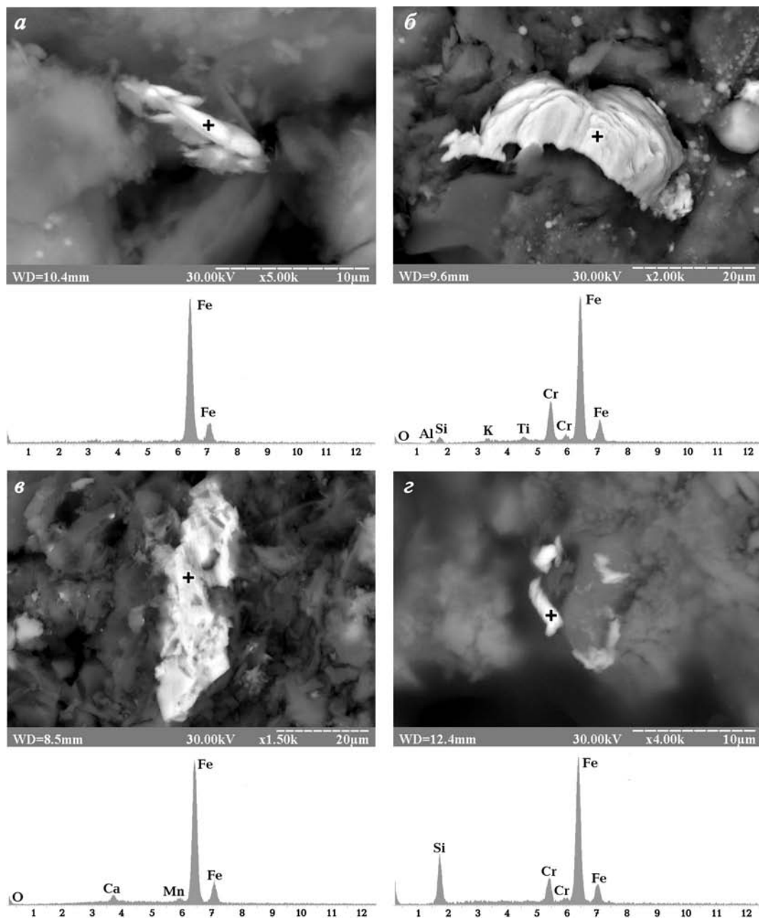
Рис. 3. Самородное железо (а), Cr-железо (б, в) и силицид железа (г) в инъекциях ТППВ по стилолитизированным трещинам флюидоразрыва в верхнемеловых известняках (Равнинный Крым, площадь Северная, скв. 2, 2722-2729 м)
