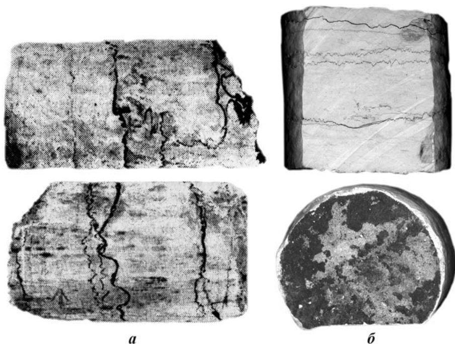
Рис. 1. Инъекции ТППВ по стилолитизированным трещинам естественного флюидоразрыва в известняках верхнего мела: а – Равнинный Крым, площадь Северная, скв. 2, 1396-1403 м; б – северо-западный шельф Черного моря, поднятие Сельского, скв. 40, 2572-2581 м
