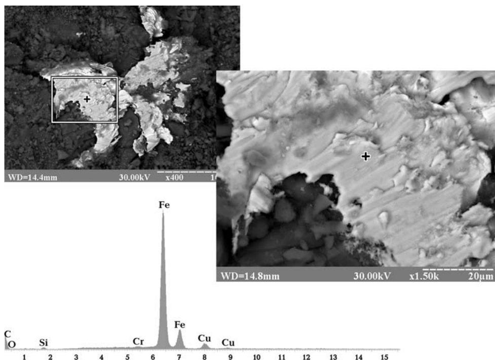
Рис. 18. Самородное железо (с примесью хрома и меди) в песчаном коллекторе-метасоматите (нефтяное месторождение Субботина, скв. 1, 2490,2–2495,8 м)
