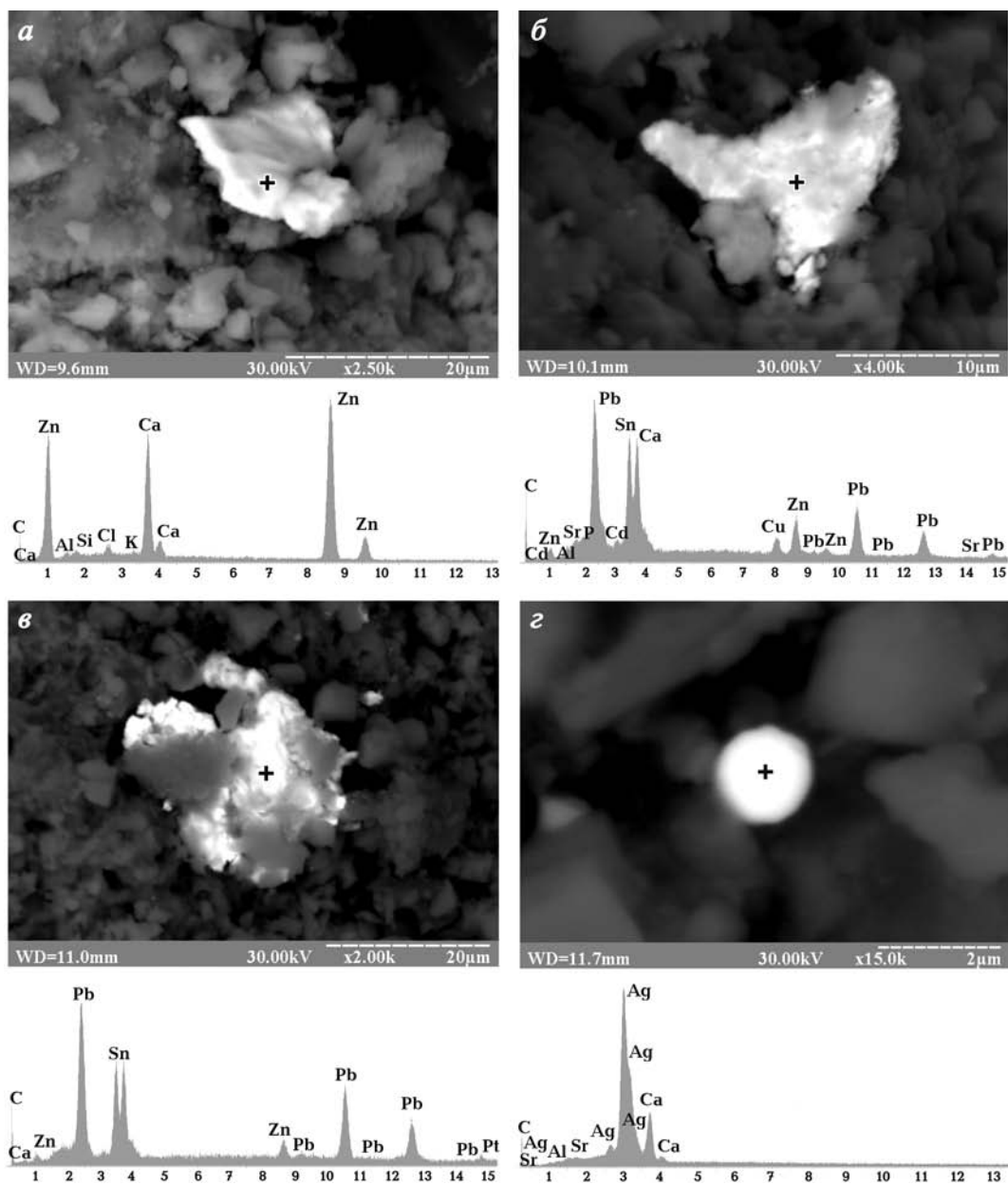
Рис. 7. Самородный цинк (а), сросток частиц самородных свинца, олова и цинка (с примесью кадмия) (б), агрегат самородных свинца, олова и цинка (в), самородное серебро (г) в гераклите
