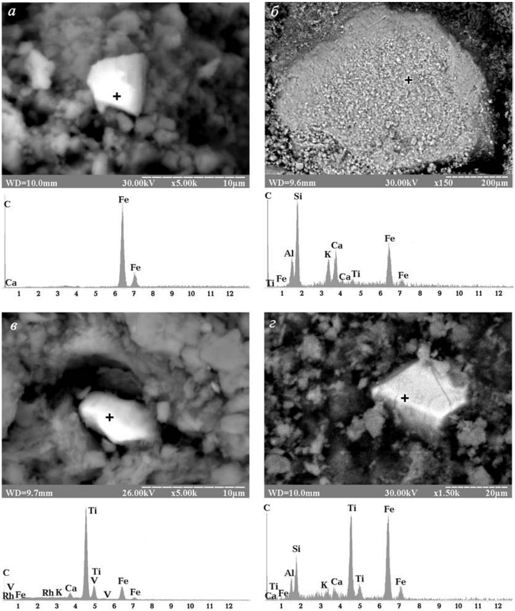
Рис. 9. Карбиды и силициды в геркците: а – карбид железа (цементит Fe_3C ?); б – муассанит (SiC) с примесью карбидов железа, кальция, титана (в остатке после кислотной обработки); в – хамрабаевит ((Ti, V, Fe)C) с примесью родия (в остатке после кислотной обработки); з – кубооктаэдрический кристалл карбида титана и железа (Ti, Fe)C (?) с характерными трещинами (в остатке после жесткой кислотной обработки)
