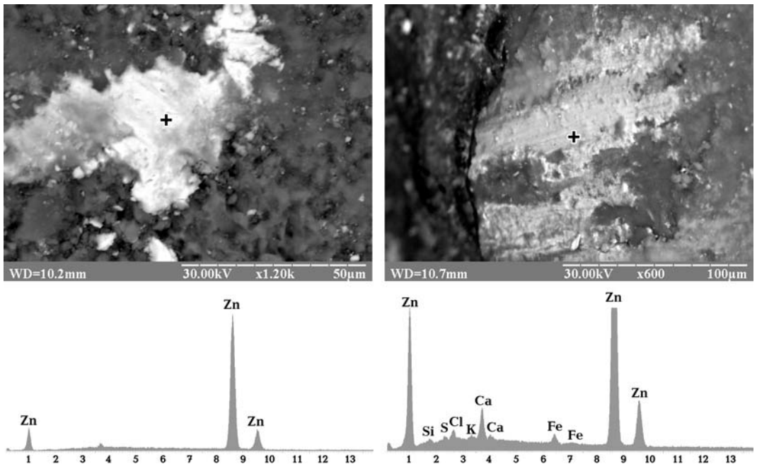
Рис. 15. Самородный цинк в барит-карбонатной корке (твердая часть) (грязевый вулкан Двуреченский, прогиб Сорокина, Черное море)
