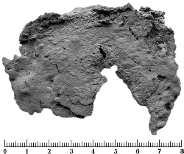
Рис. 13. Литифицированная пористая корка (фумарольное образование) (грязевый вулкан Двуреченский, прогиб Сорокина, Черное море)
