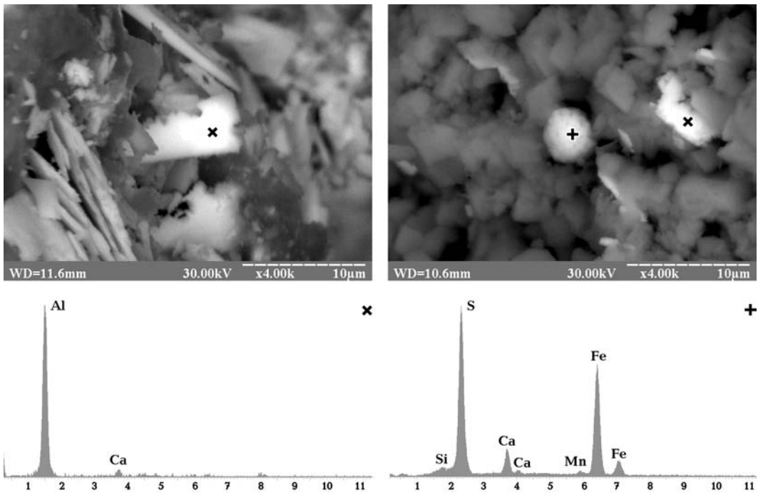
Рис. 16. Самородный алюминий (и фрамбоидальный пирит) в кальцит-арагонитовой корке (рыхлая часть) (грязевый вулкан Двуреченский, прогиб Сорокина, Черное море)
