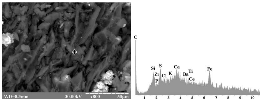
Рис. 2. Микроструктура и рентгеновский спектр ТППВ – Равнинный Крым, площадь Северная, скв. 2, 2587-2594 м (микроскоп РЭМ-106 с рентгеноспектральным зондом, ЧО УкрГГРИ)
