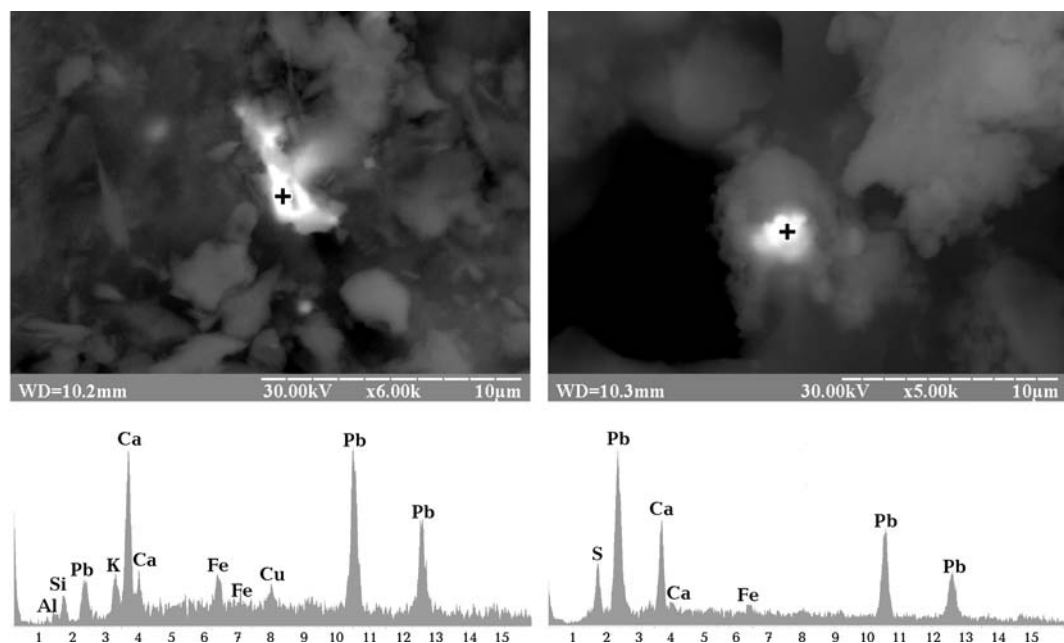
Рис. 4. Самородный свинец в инъекциях ТППВ по стилолитизированным трещинам флюидоразрыва в верхнемеловых известняках (Равнинный Крым, площадь Северная, скв. 2, 2587-2594 м)
