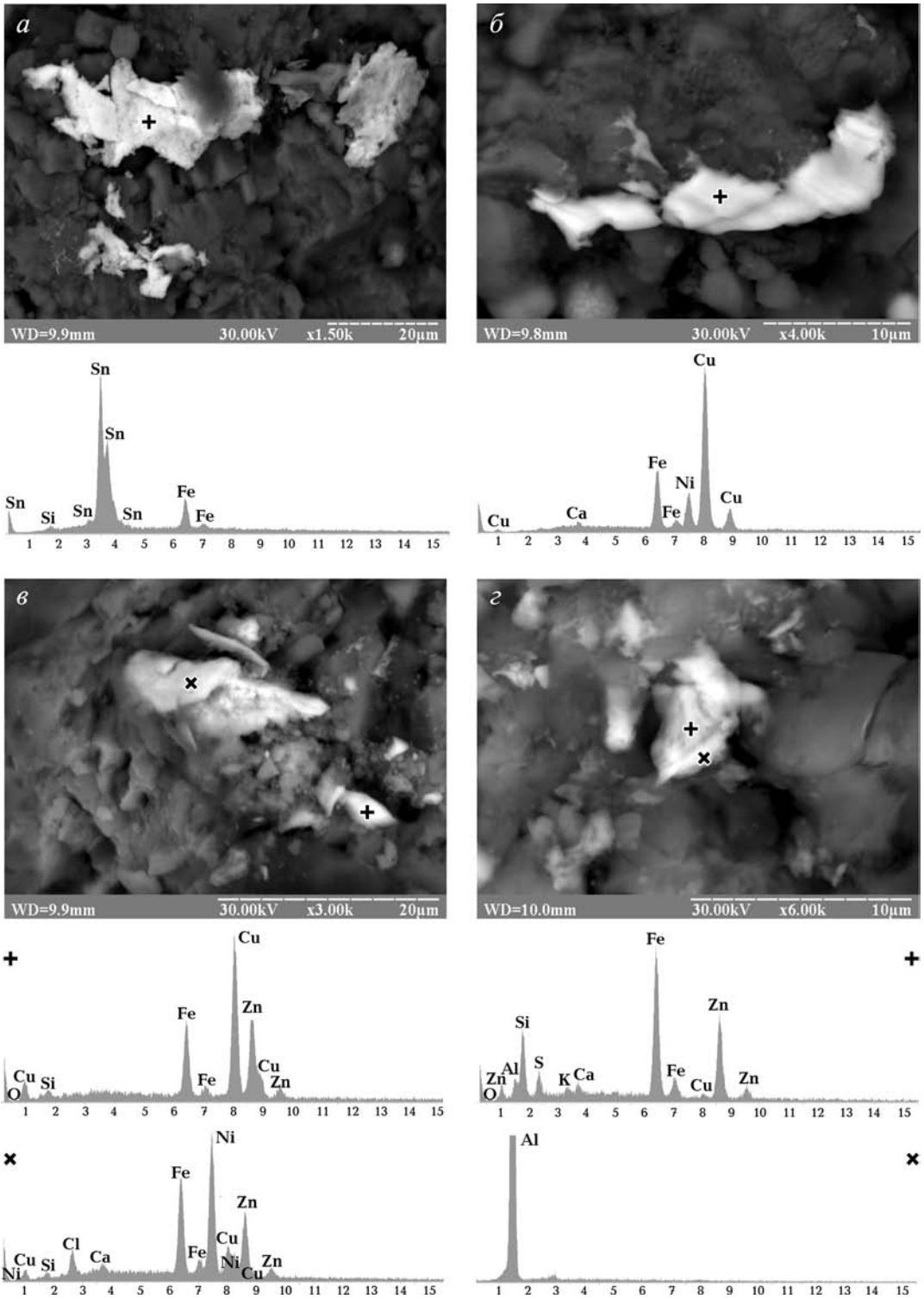
Рис. 10. Самородные металлы и природные сплавы в взрывной бомбе (грязевый вулкан Карабетова гора, Таманский п-ов, извержение 29.07.2005 г., коллекция В.А. Алексеева): а – самородное олово и железо; б – природный сплав меди с железом и никелем; в – природные сплавы железа с никелем и меди с цинком (латунь); г – сросток самородных железа, цинка и алюминия
