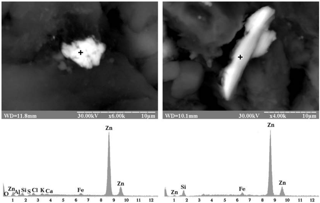
Рис. 20. Самородный цинк в песчаном коллекторе-метасоматите (нефтяное месторождение Субботина, скв. 1, 2490,2–2495,8 м)
