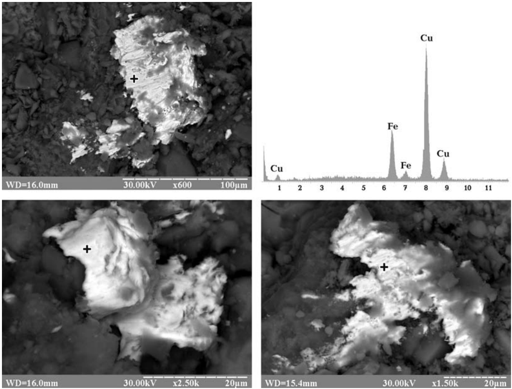
Рис. 19. Самородная медь с примесью железа в песчаном коллекторе-метасоматите (нефтяное месторождение Субботина, скв. 1, 2490,2–2495,8 м)
