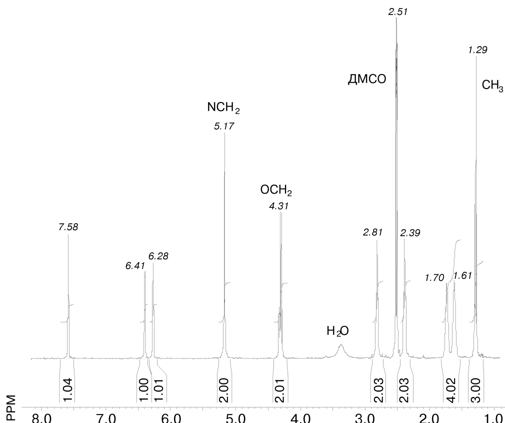
Рис. 1. Спектр ЯМР ^1\text{H} етилового ефіру 1-фурфурил-2-оксо-4-гідрокси-1,2,5,6,7,8-гексагідрохінолін-3-карбонової кислоти (7) - сигнал протону 4-ОН-групи при 13,35 м.д. за браком місця не наведено.
