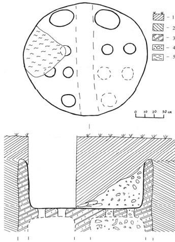
Мал.1. Схематичний план досліджених решток горна Диканька, Полтавщина. Середина XVIII ст. (?). 1: сіро-чорний ґрунт з окремими знахідками XIX-XX століть; 2: жовто-бурий материковий суглинок; 3: прожарений суглинок стінок та череня посудної камери; 4: заповнення посудної камери горна зі значними включеннями перепаленої глини та фрагментів гончарний виробів; 5: перекоп 1920 – 1940-х років. Малюнок Анатолія Щербаня
