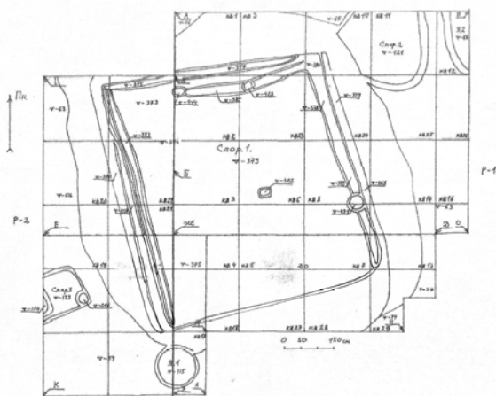
Рис. 5. План котловану флігеля палацового комплексу на Гончарівці по матеріку
