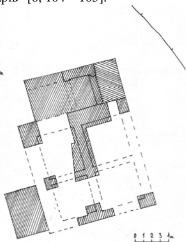
Рис. 4. План палацу Івана Мазепа на Гончарівці за наслідками досліджень 1995 – 2010 рр.
