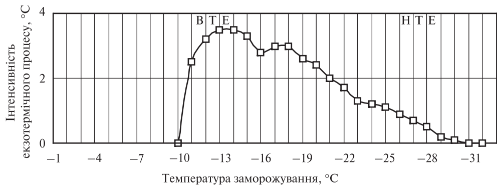
Рис. 5. Екзотерми льодоутворення однорічних пагонів M. salicifolia
