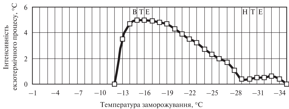
Рис. 4. Екзотерми льодоутворення однорічних пагонів M. kobus
