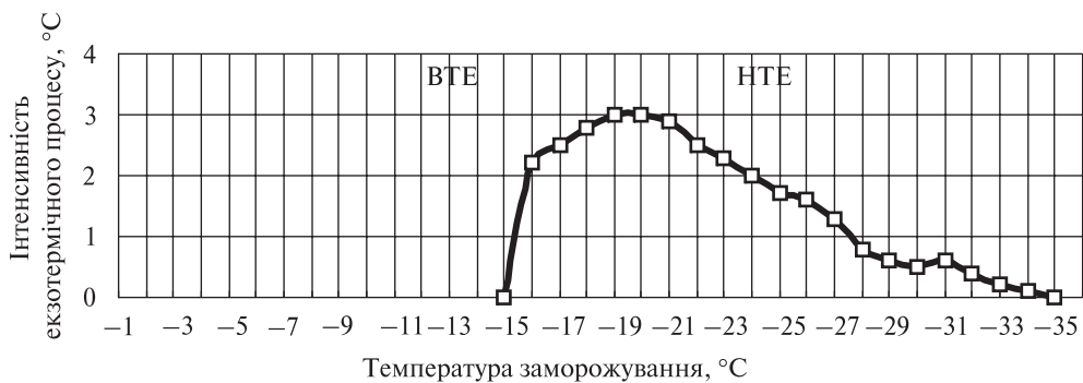
Рис. 2. Екзотерми льодоутворення однорічних пагонів M. denudata Fig. 2. Exotherms of ice formation of M. denudata annual shoots
