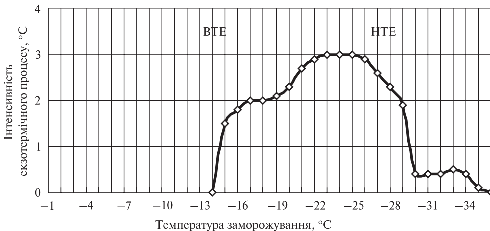
Рис. 3. Екзотерми льодоутворення однорічних пагонів M. × soulangiana Fig. 3. Exotherms of ice formation of M. x soulangiana annual shoots
