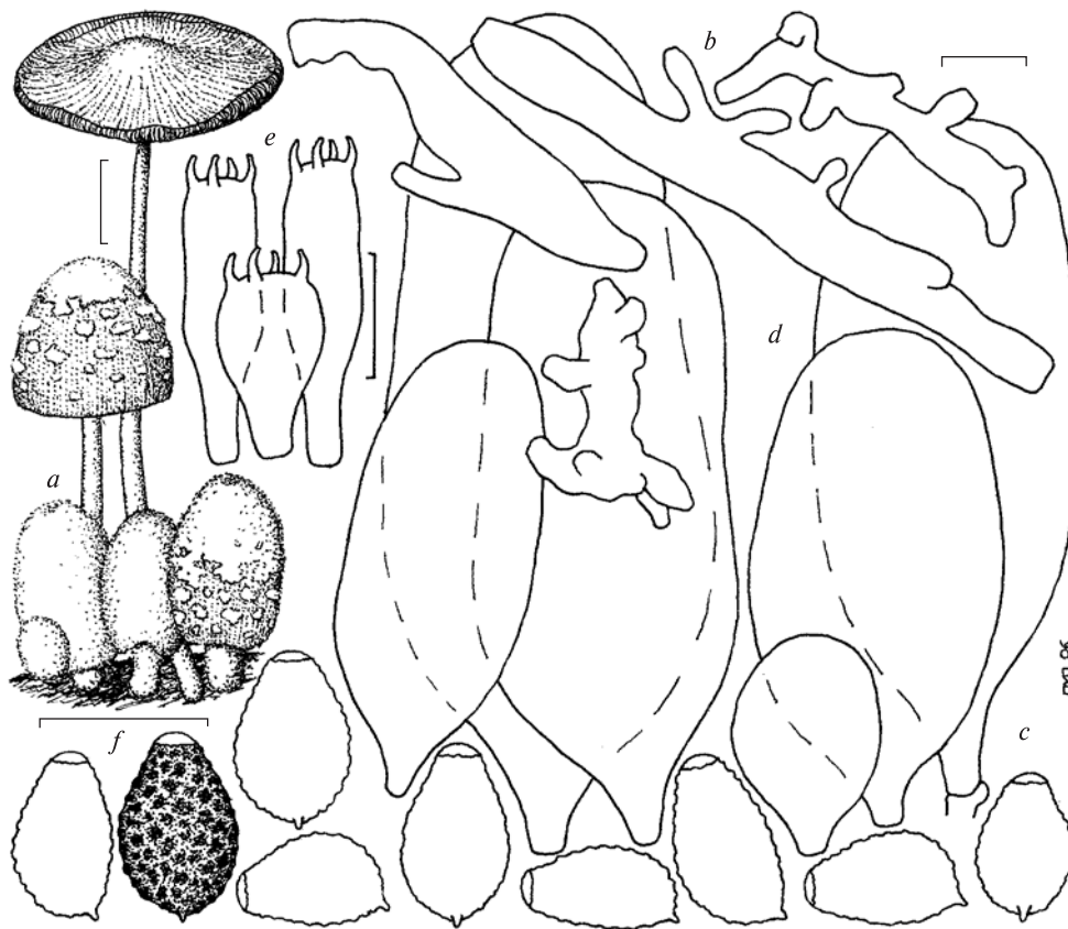
Рис. 1. Coprinus echinosporus Buller: a — плодові тіла, b — елементи покривала, c — хейлоцистиди, d — плевроцистиди, e — базидії, f — спори. Тут і на рисунках 3, 4: масштабна лінійка для плодових тіл = 1 см, для мікроструктур = 10 мкм
