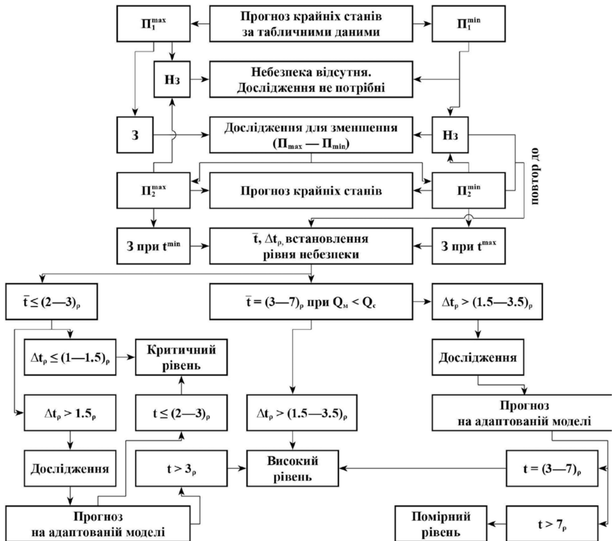
Рис. 2. Схема визначення рівня небезпеки від нафтопродуктового забруднення P_1^{\max} — початкові параметри, що прискорюють пересування НП; P_1^{\min} — початкові параметри, що уповільнюють пересування НП; P_2^{\max} , P_2^{\min} — уточнені параметри; Z > ГДК — забруднення; H_3 < ГДК — відсутність забруднення; t — термін забруднення; t^{\max} , t^{\min} — максимальний, мінімальний терміни забруднення; \bar{t} — середньоарифметичний термін забруднення; \Delta t_p — імовірна похибка терміну забруднення; Q_m , Q_c — вартість моніторингу та санаційних робіт.
