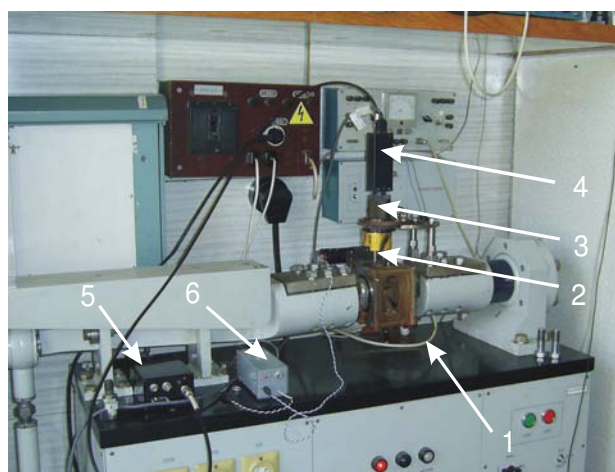
Рис. 2. Загальний вигляд установки: 1 – випробувальна машина циклічного згину; 2 – освітлювач; 3 – вузол оптичних елементів; 4 – камера SONY XCD-SX910; 5 – давач положення; 6 – блок стабілізованого живлення
