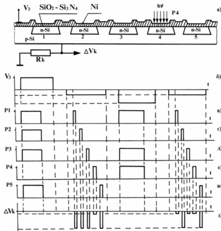
Рис. 1. а) Поперечний переріз ПООП на основі багатофункціональних фоточутливих елементів - лінійки інтегральних МНОН-п-р структур;
