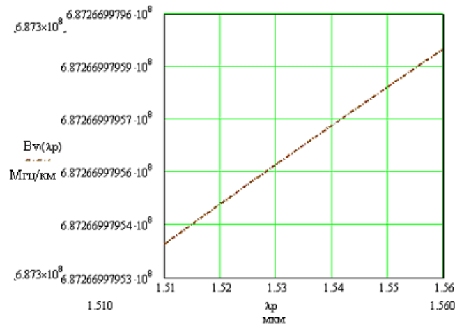
Рис.13.Смуга пропускання оптичного волокна MMF 400/1000мкм
