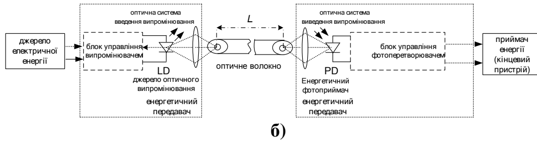
Рис.7. Загальні структури волоконно-оптичних каналів: а) – інформаційного; б) – енергетичного
