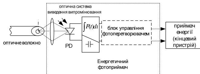
Рис.8 . Енергетичний фотоприймач з інтегратором прийнятої потужності
