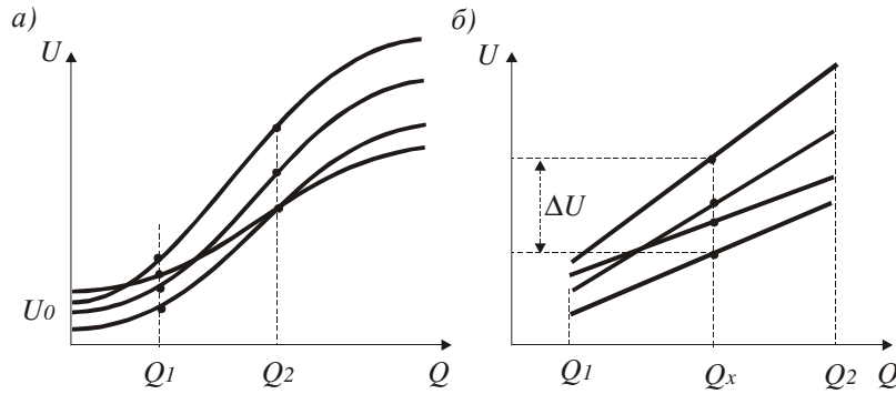
Рис. 5. Статичні характеристики спектрофотометра з горизонтальним атомізатором (а) та градуювальні (б).
