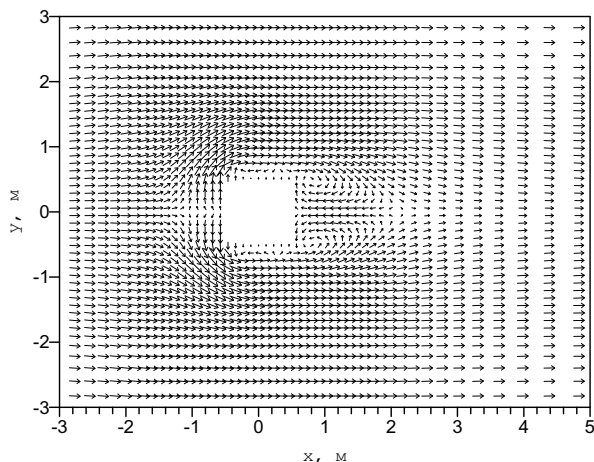
Рис.2. Рассчитанное поле скорости для условий эксперимента [7]
