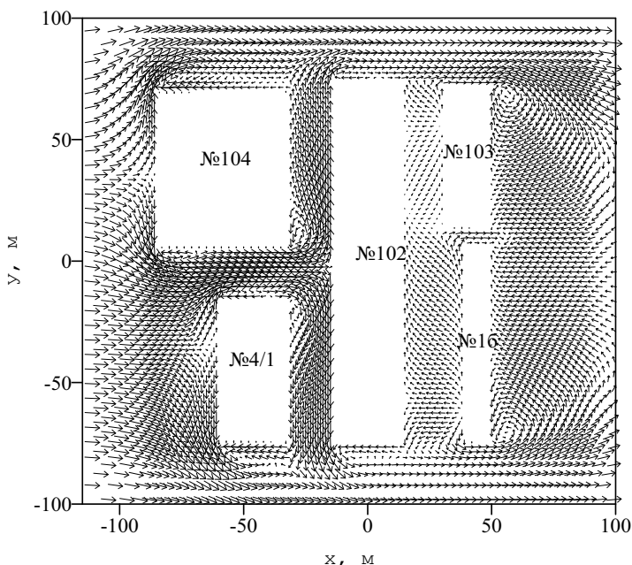
Рис.3. Рассчитанное приземное поле ветра вокруг зданий на промплощадке ПХЗ, розраховане моделлю DETATOX (показаны векторы в каждом шестом узле)
