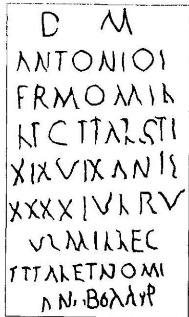
Рис. 3. Прорисовка епітафії
