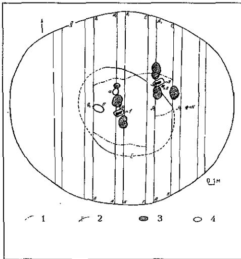
Рис. 3. Загальний план кургану № 2 біля с. Журавлиха: 1 — межа підрізки материка; 2 — контур 1-го і 2-го насипів; 3 — викид; 4 — яма
