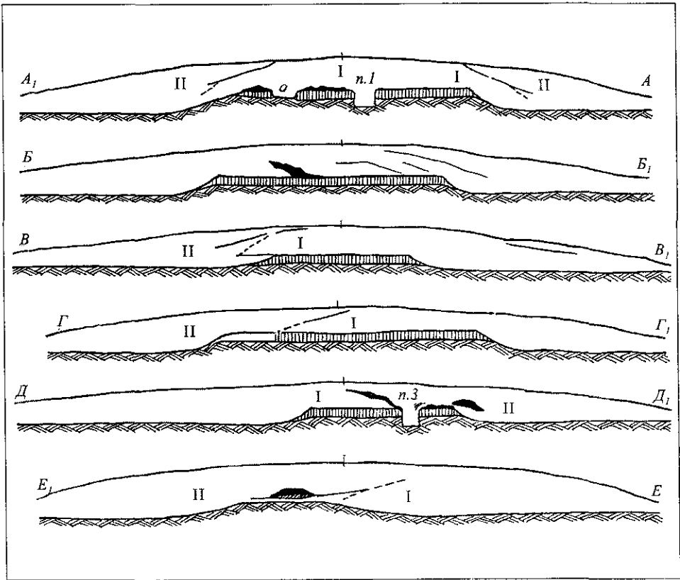
Рис. 4. Профілі кургану № 2 біля с. Журавлиха. Умовні позначення див. рис. 2
