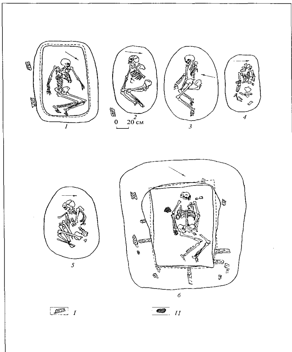
Рис. 7. Поховання з кургану № 3 біля с. Журавлиха. Плани поховань: 1 — № 4, 2 — № 5, 3 — № 6, 4 — № 7, 5 — № 1; 6 — № 2; I — дерево; II — червона фарба
