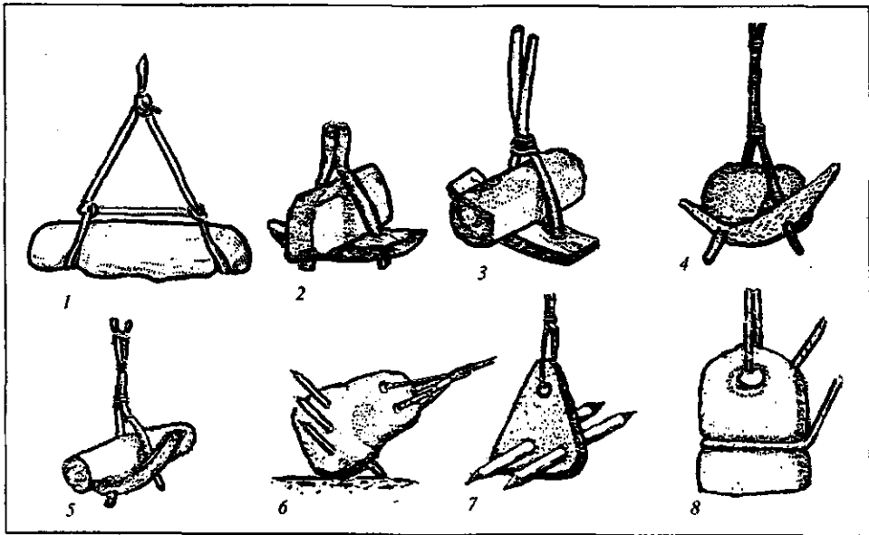
Рис. 4. Зразки кам'яних якорів: 1 — кобаківська культура; 2—5 — знахідки з різних частин світу; 6 — Середземне море; 7 — Єгипет (1 — за Е.С. Шарафутдиновом; 2—7 — за Л.Н. Скрягиним)
