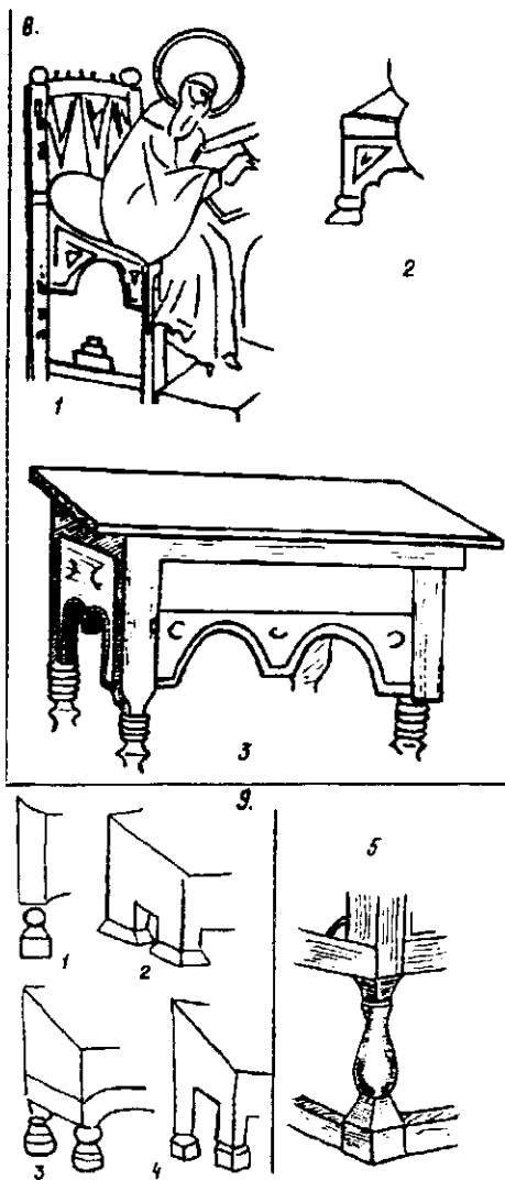
Рис. 8. Лиштва у вигляді арки і різьблення на меблях: 1 — фрески Кирилівської церкви у Києві; 2 — мініатюра Радзивілівського літопису; 3 — пізніша аналогія: столик російської роботи XVII ст.
