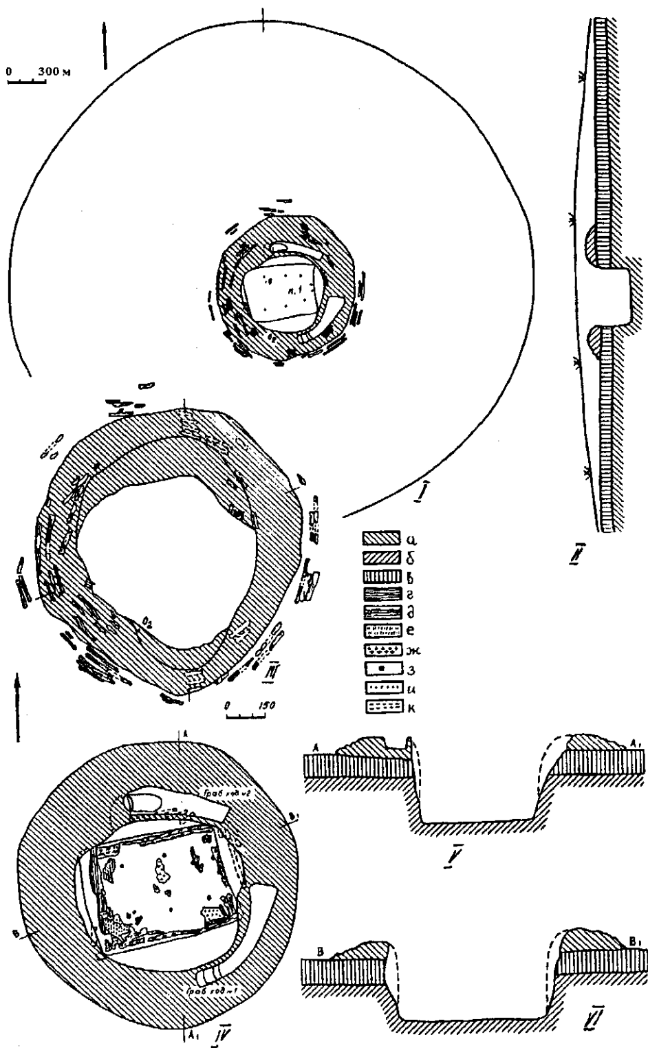
Рис. 7. Іванівка, курган 5. I—II — план та профіль кургану; III — надмогильна конструкція із залипками дерева; IV—VI — план та розрізи поховальної споруди; а — глина материкового викиду; б — материк; в — поховальний ґрунт; г — дерево; д — обпалене дерево; е — кора; ж — ділянки перекриття з обпаленою глиною; з — стовпові ями; и — грабіжницький хід; к — дерев'яні плахи під валом.
