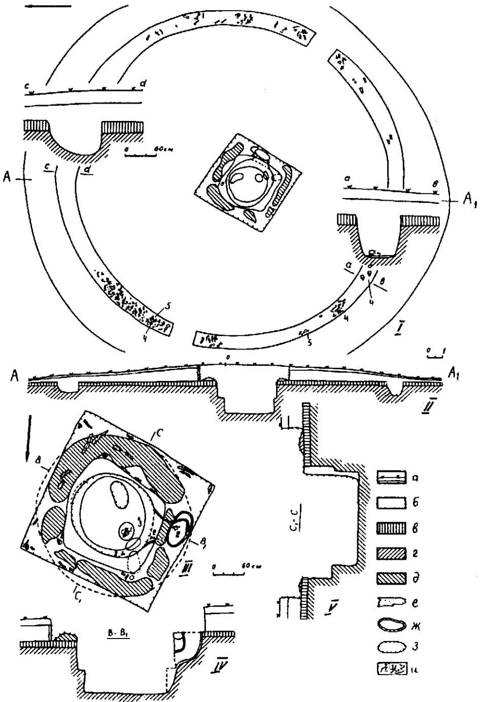
Рис. 2. Іванівка, курган 3. I—II — план та профіль кургану; III—V — план та розрізи поховальної споруди; а — орний шар; б — чорноземний насип; в — поховальний ґрунт; г — материк; д — глина могильного викиду; е — дерево; ж — давній грабіжницький лаз; и — кістки тварин. 1 — схованка; 2 — фрагменти панцирного набору; 3 — панцирні платівки; 4 — людські кістки; 5 — уламки амфори.
