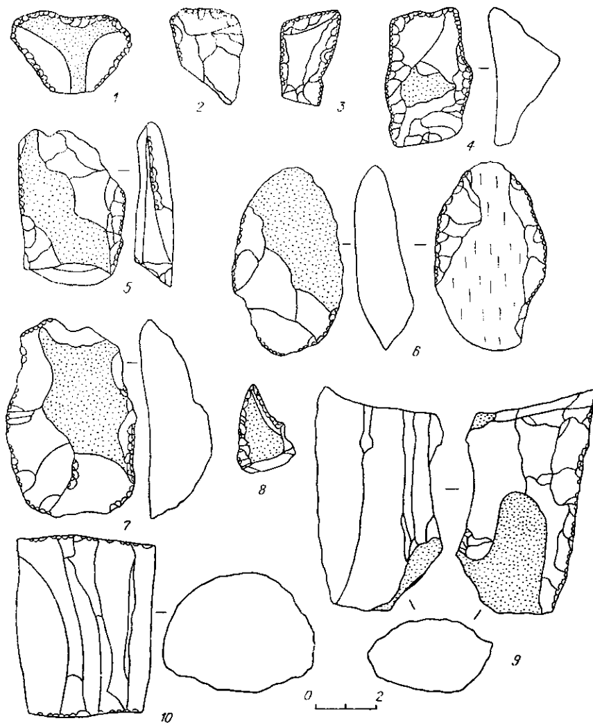
Рис. 4. Хут. Коник. Крем'яні вироби (1—10)
