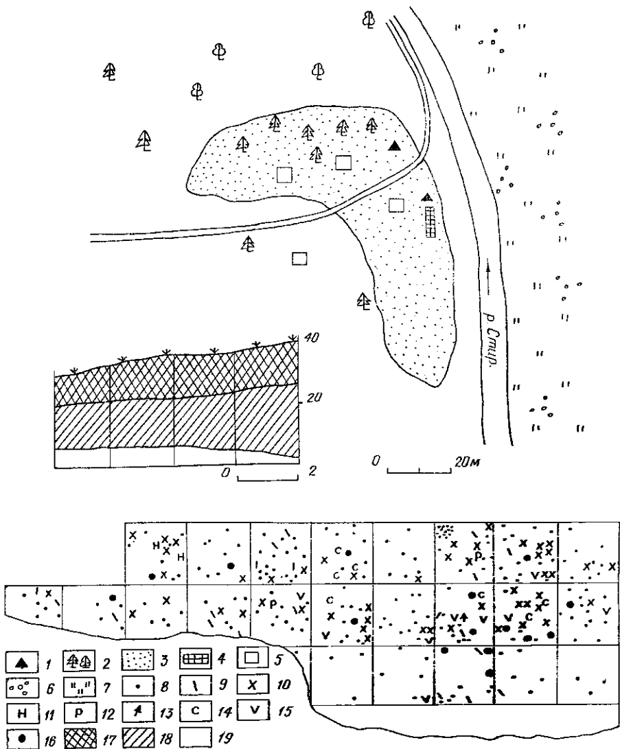
Рис. 1. Плани розміщення неолітичного поселення Коник та розкопок на ньому: 1 — поселення, 2 — ліс, 3 — дюна, 4 — розкоп, 5 — двір, 6 — чагарник, 7 — луг, 8 — відщеп, 9 — пластина, 10 — кераміка, 11 — нуклеус, 12 — різець, 13 — наконечник, 14 — скребок, 15 — пластина з ретушю, 16 — відщеп з ретушю, 17 — ґрунт, 18 — підґрунтя, 19 — материк
