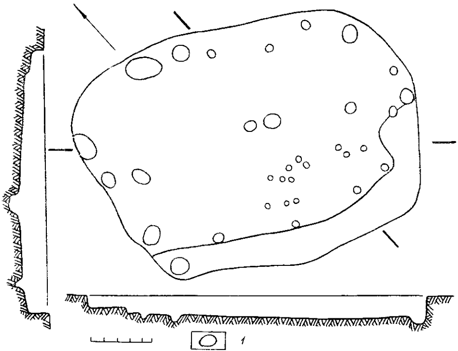
Рис. 1. План та розрізи житла 5.
